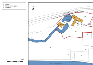
Plan-masse et de situation, section AB. Dess. Mathias Papigny IVR43_20142501902NUDA
