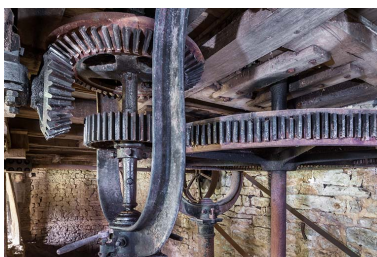
Détail des engrenages du beffroi de moulin. Phot. Jérôme Mongreville IVR43_20142501174NUC4A
