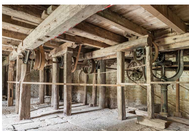
Vue d'ensemble de l'étage de soubassement. Phot. Jérôme Mongreville IVR43_20142501173NUC4A
