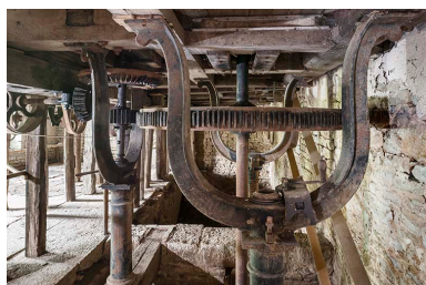
Etage de soubassement. Beffroi du moulin. Phot. Jérôme Mongreville IVR43_20142501175NUC4A
