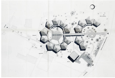
Plan des toitures. 20 janvier 1978. Phot. Jérôme Mongreville, Autr. Mestoudjian K. I. (architecte), Autr. Moryusef P. (architecte), Autr. Solère G. (architecte) IVR43_20112500243NUC4A
