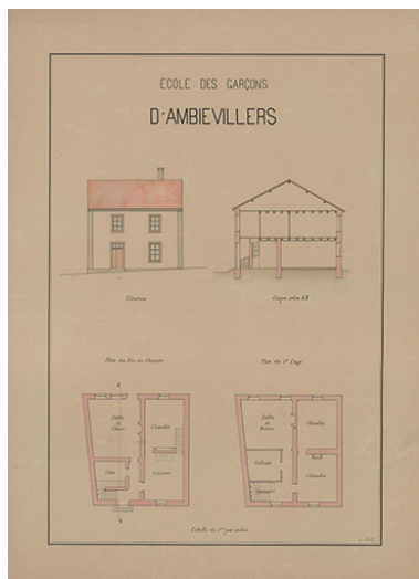
Plan de l'école des garçons : élévation, coupe, plan du rez- de-chaussée, plan du 1er étage. IVR43_20167000012NUC4A
