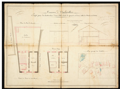
Projet pour la construction d'une salle d'école des garçons et d'une salle de mairie. Phot. Sonia Dourlot, Autr. Pierre Mougenot IVR43_20167000011NUC4A
