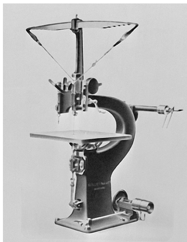
Scie alternative à découper pour bois et métaux munie d'une perceuse. Phot. Yves Sancey IVR43_20022500921X
