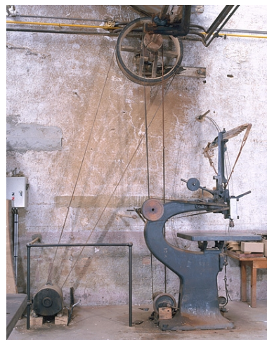
Vue d'ensemble depuis l'ouest, avec le moteur électrique et son système d'entraînement. Phot. Yves Sancey IVR43_20022500757XA
