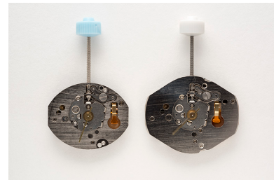
2 modules de montre à quartz France Ebauches FE 5120 et 6120 (côté cadran). Phot. Sonia Dourlot IVR43_20152502573NUC4A
