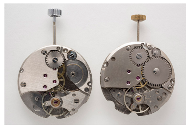
2 mouvements de montre mécaniques France Ebauches FE 140-1 et 140-2A (côté ponts). Phot. Sonia Dourlot IVR43_20152502548NUC4A
