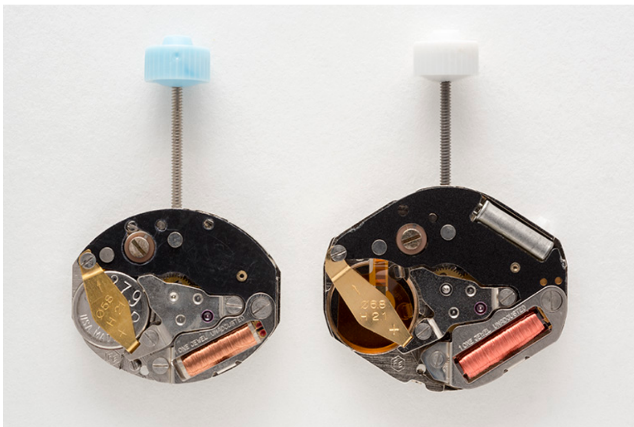
2 modules de montre à quartz France Ebauches FE 5120 et 6120 (côté ponts).
