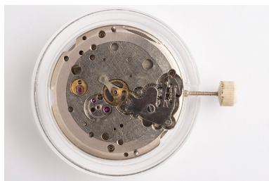
Mouvement de montre mécanique France Ebauches FE 140 (côté cadran). Phot. Sonia Dourlot IVR43_20152500006NUC4A
