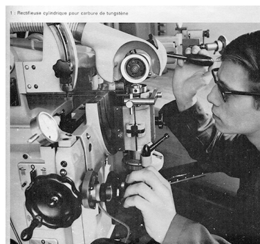
France Ebauches, une haute technicité. 1. Rectifieuse cylindrique pour carbure de tungstène, 1970. IVR43_20182501550NUC4A
