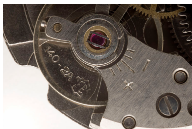
Mouvement de montre mécanique France Ebauches FE 140-2A : logotype de la société et indication du modèle. Phot. Sonia Dourlot IVR43_20152502553NUC4A
