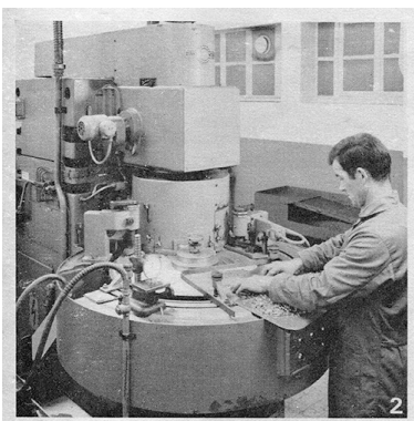
France Ebauches, une haute technicité. 2. Machine à surfer de très haute précision, 1970. IVR43_20182501551NUC1A
