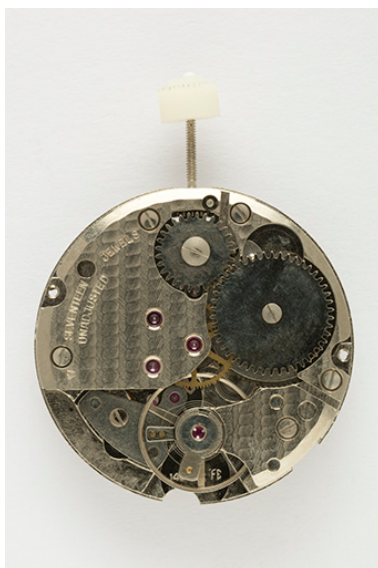
Mouvement de montre mécanique France Ebauches FE 140-C (côté ponts). Phot. Sonia Dourlot IVR43_20162500743NUC4A
