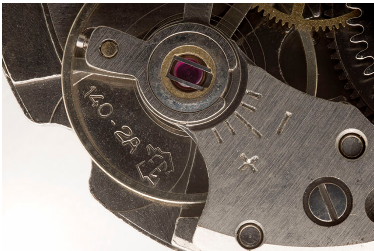
Mouvement de montre mécanique France Ebauches FE 140-2A : logotype de la société et indication du modèle.
