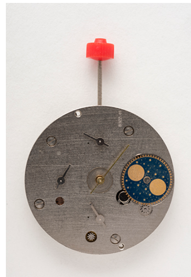
Module de montre à quartz France Ebauches FE 11500. Phot. Sonia Dourlot IVR43_20152502570NUC4A
