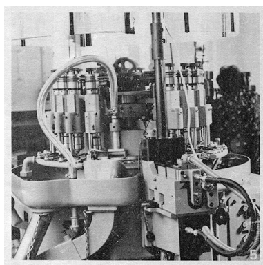
France Ebauches, une haute technicité. 5. Machine à percer multiple à charge automatique, 1970. IVR43_20182501554NUC1A
