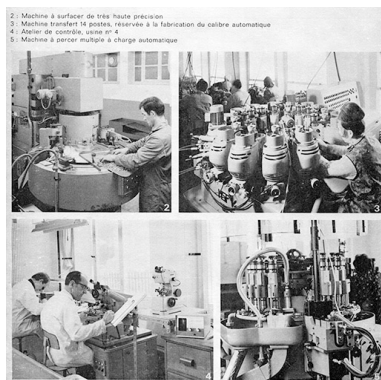
France Ebauches, une haute technicité. [2 à 5. Intérieurs d'ateliers (avec machines à surfer, à percer et machine transfert), celui de contrôle dans l'usine Anguenot de Villers-le-Lac (vue n° 4)], 1970. IVR43_20192500564NUC4A
