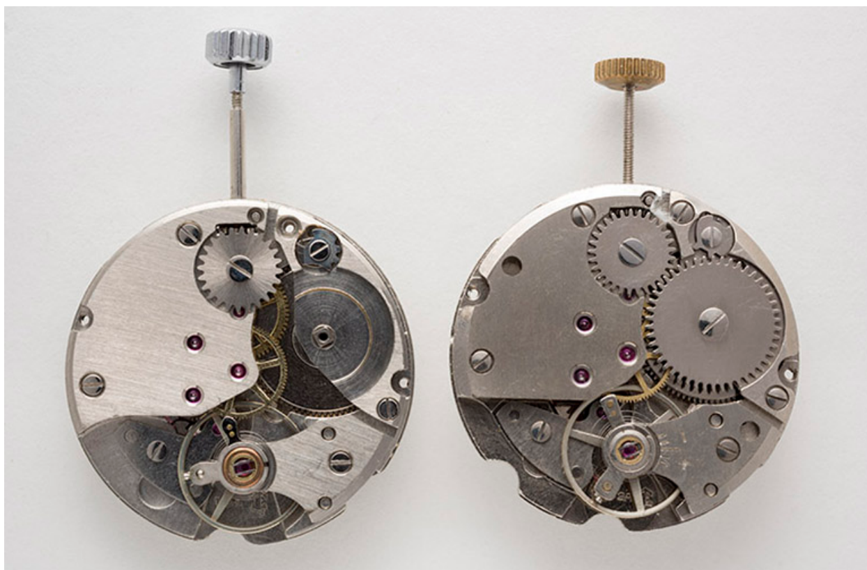
2 mouvements de montre mécaniques France Ebauches FE 140-1 et 140-2A (côté ponts).
