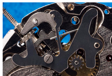
Mouvement de montre mécanique France Ebauches FE 233-68-E-21 : la tirette. Phot. Sonia Dourlot IVR43_20162500755NUC4A
