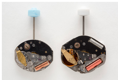
2 modules de montre à quartz France Ebauches FE 5120 et 6120 (côté ponts). Phot. Sonia Dourlot IVR43_20152502574NUC4A
