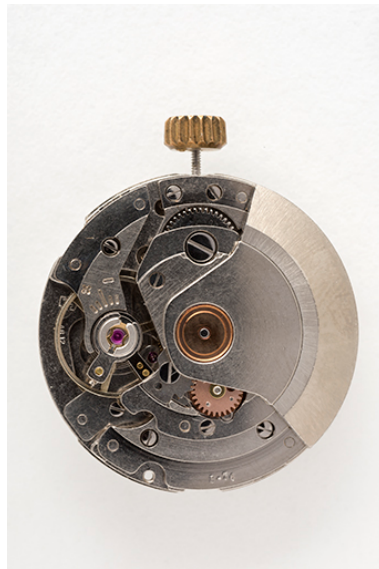
Mouvement de montre mécanique France Ebauches FE 4612 (côté ponts). Phot. Sonia Dourlot IVR43_20152502556NUC4A
