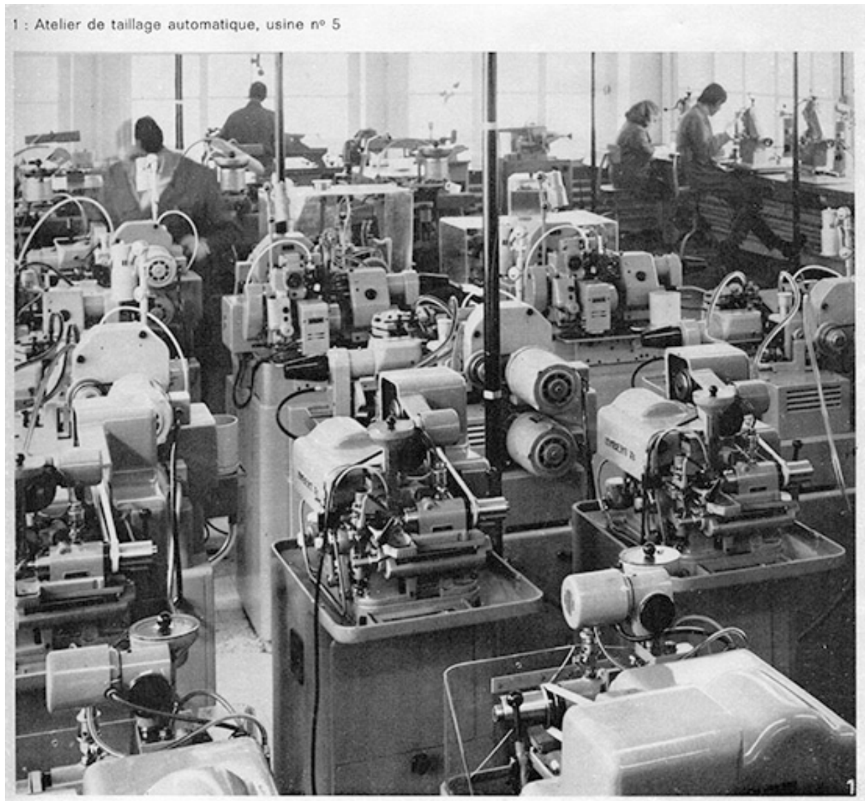
France Ebauches, des moyens modernes. 1. Atelier de taillage automatique, usine n° 5 [Cupillard à Villers-le-Lac], 1970.
