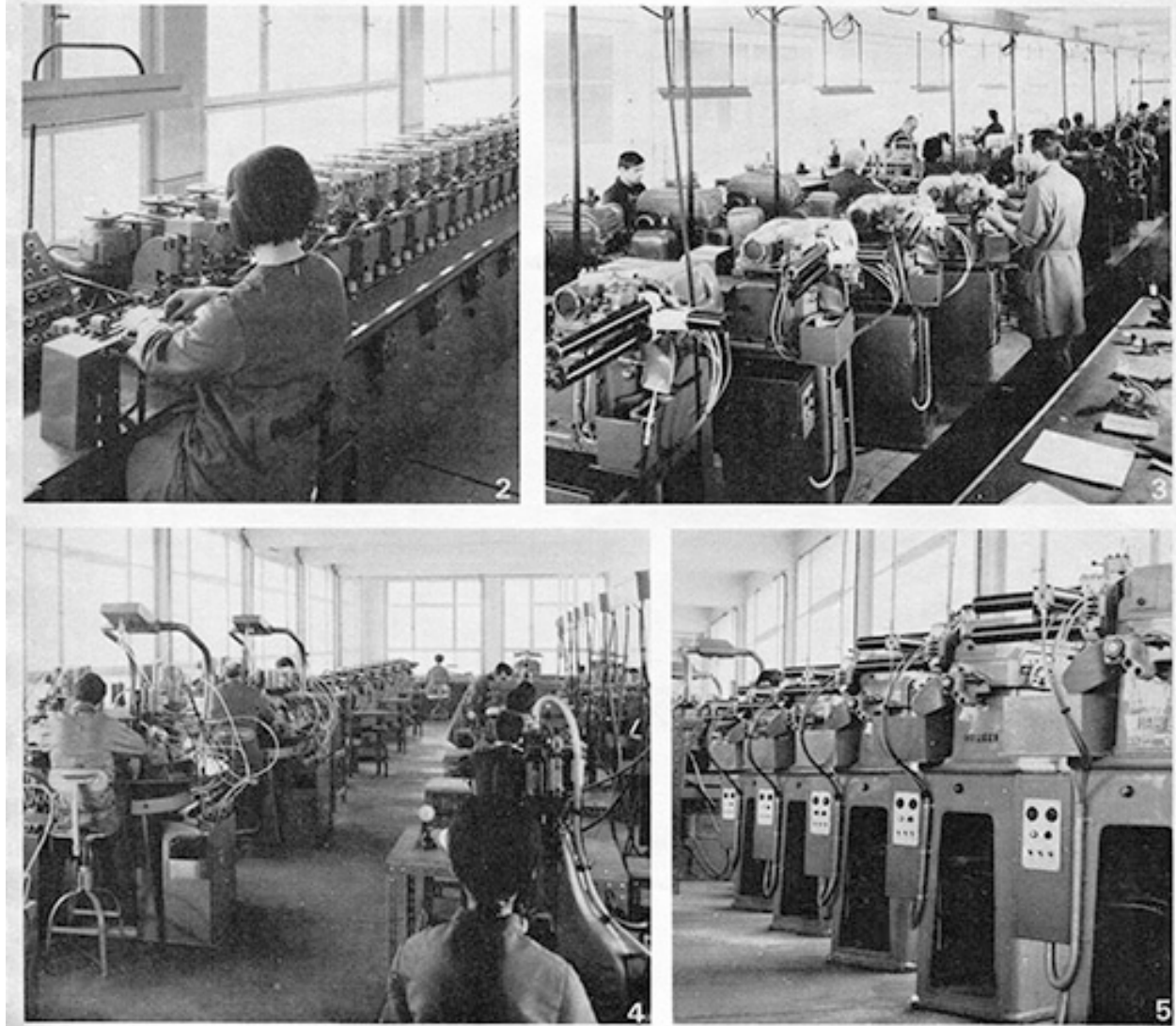
2 : Transfert linéaire France Ebauches 3 : Vue générale d'un atelier, usine n° 4 4 : Vue générale d'un atelier, usine n° 2 5 : Batterie de machines à contourner automatiques
