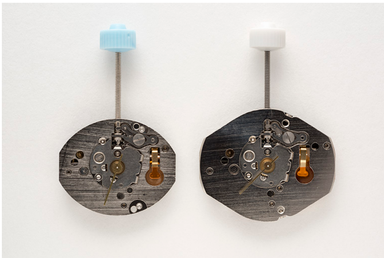
2 modules de montre à quartz France Ebauches FE 5120 et 6120 (côté cadran).
