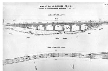
Viaduc de la grande Roche à 7 arches de 10,00 m d'ouverture, surbaissées. Plan d'ensemble [et] Elévation aval, [1919]. Phot. Jérôme Mongreville IVR43_20003900867X
