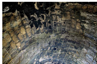
Tunnel du Champ de Bienne : détail de la voûte.
