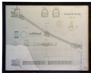
Conduite forcée [plan, coupes et élévation], 1908. Phot. Yves Sancey, Autr. Société des Forces motrices de l'Est IVR43_20122502133NUC2A
