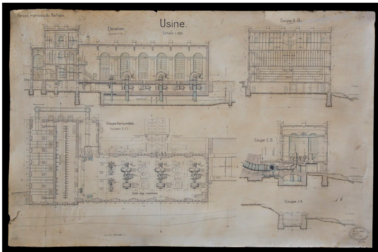
Forces motrices du Refrain. Usine [plan au rez-de-chaussée et coupes longitudinale et transversales], 1908.
