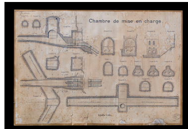
Société des Forces motrices du Refrain. Plan d'exécution. Chambre de mise en charge [plan et coupes], 1908. Phot. Yves Sancey, Autr. Société des Forces motrices de l'Est IVR43_20122502166NUC2A
