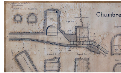
Société des Forces motrices du Refrain. Plan d'exécution. Chambre de mise en charge [détail : coupe longitudinale], 1908. Phot. Yves Sancey, Autr. Société des Forces motrices de l'Est IVR43_20122502167NUC2A
