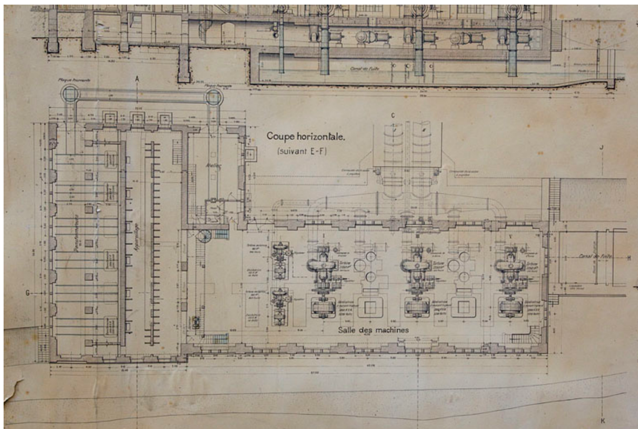
Forces motrices du Refrain. Usine [détail : plan au rez-de-chaussée], 1908.
