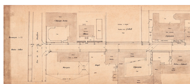
Plan-masse de l'usine (partie sud), s.d. [vers 1920]. IVR43_20192500747NUC4A
