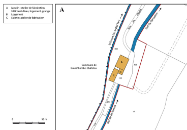
Plan-masse et de situation. Extrait du plan cadastral, 2016, section A, 1/2 500 agrandi à 1/1 000. Dess. Bertrand Turina IVR43_20182501337NUDA
