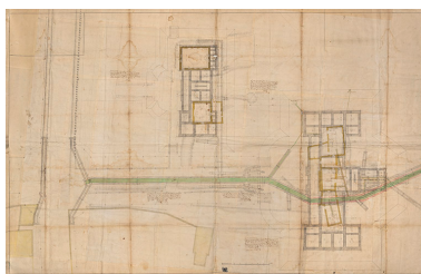
Projet d'aménagement du secteur du canal situé au nord de la Fosse Pageot (1761). Repro. Jérôme Mongreville, Autr. Jean Querret
