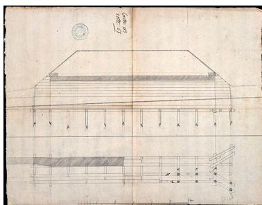
Plan et coupe longitudinale du ponceau de la chaussée de l'étang (vers 1761). Phot. Jérôme Mongreville, Autr. Jean Querret IVR43_20207000023NUC4A
