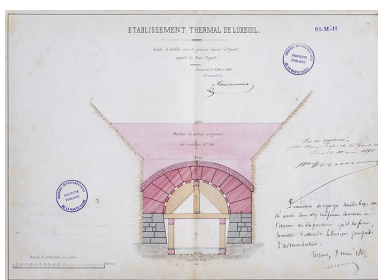
Projet de reconstruction de la voûte du tunnel du canal dit Fosse Pageot (1865). Phot. Jérôme Mongreville, Autr. Félix-Hercule Grandmougin IVR43_20207000454NUC4A
