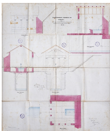
Projet de construction d'un lavoir couvert (1862). Phot. Jérôme Mongreville, Autr. Félix-Hercule Grandmougin IVR43_20207000453NUC4A
