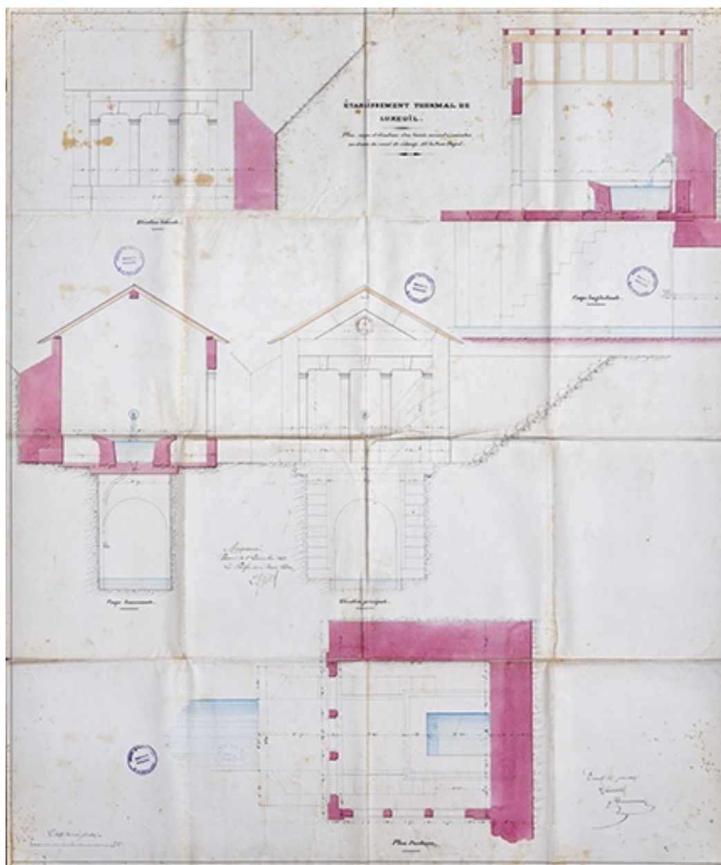
Projet de construction d'un lavoir couvert (1862).
