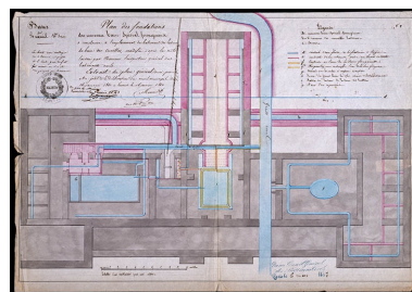
Tracé du canal dans les fondations du bâtiment nord dit du Grand Bain. Repro. Jérôme Mongreville, Autr. Charles-Antoine Monnier IVR43_20207000436NUC4A
