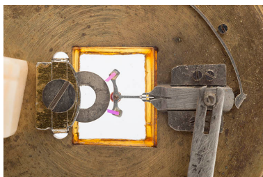
Vue de détail de l'outil. De gauche à droite : la rondelle et sa fixation, l'ancre (dont les deux palettes sont en appui contre la rondelle), la coulisse et son ressort. Phot. Sonia Dourlot IVR43_20152500434NUC4A
