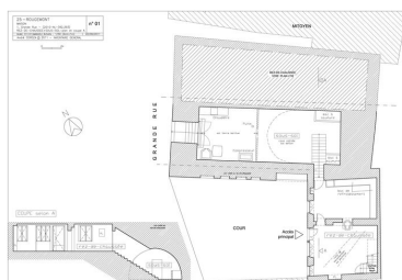
Plan et coupe A du rez-de-chaussée et du sous-sol. Dess. André Céréza IVR43_20112501110NUDYY
