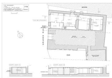
Plan et coupe B et C du rez-de-chaussée. Dess. André Céréza IVR43_20112501111NUDYY
