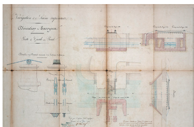
Navigation de la Saône supérieure - Dérivation de Savoyeux - Porte de garde avec pont (1843). Phot. Jérôme Mongreville, Autr. A. Voinchez IVR43_20207000111NUC4A
