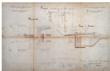
Navigation de la Saône supérieure - Dérivation de Savoyeux - Porte de garde avec pont (1843). Phot. Jérôme Mongreville, Autr. A. Voinchez IVR43_20207000109NUC4A
