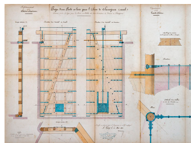
Perfectionnement de la Saône supérieure - Département de la Haute-Saône - Projet de portes en bois pour les écluses portes de garde des dérivationes de Vereux et Savoyeux (1845).
