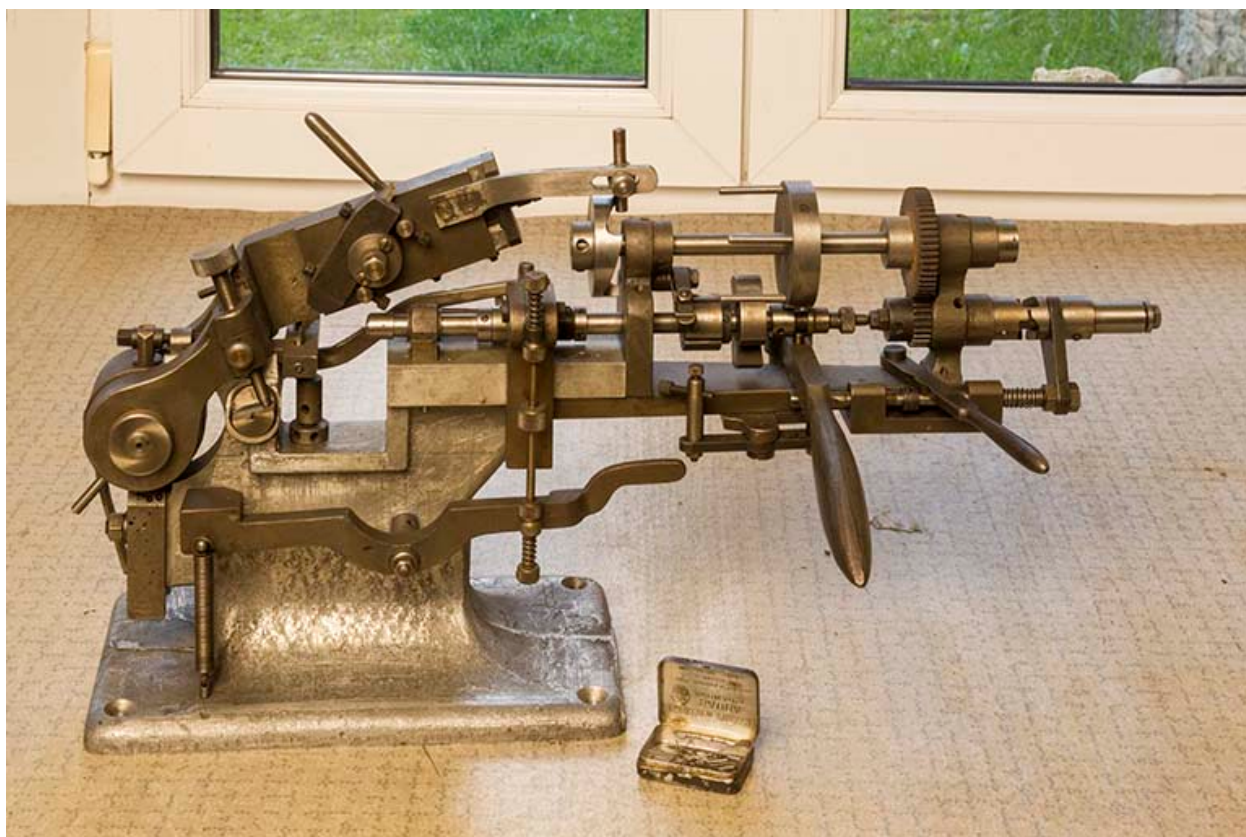
Exemple de production de l'atelier : machine à fabriquer les tire-nerfs pour dentiste.
