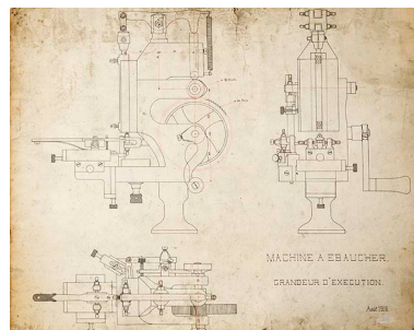
Machine à ébaucher. Grandeur d'exécution, août 1916. Phot. Yves Sancey, Autr. Adelin Berçot IVR43_20132501936NUC2A
