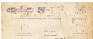
Tour à percer. Grandeur naturelle, 5 août 1912. Phot. Yves Sancey, Autr. Adelin Berçot IVR43_20132501938NUC2A
