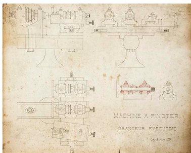
Machine à pivoter. Grandeur exécutive, septembre 1916. Phot. Yves Sancey, Autr. Adelin Berçot IVR43_20132501935NUC2A
