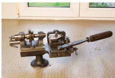
Exemple de production de l'atelier : machine à tamponner (insérer les tampons dans le cylindre).
