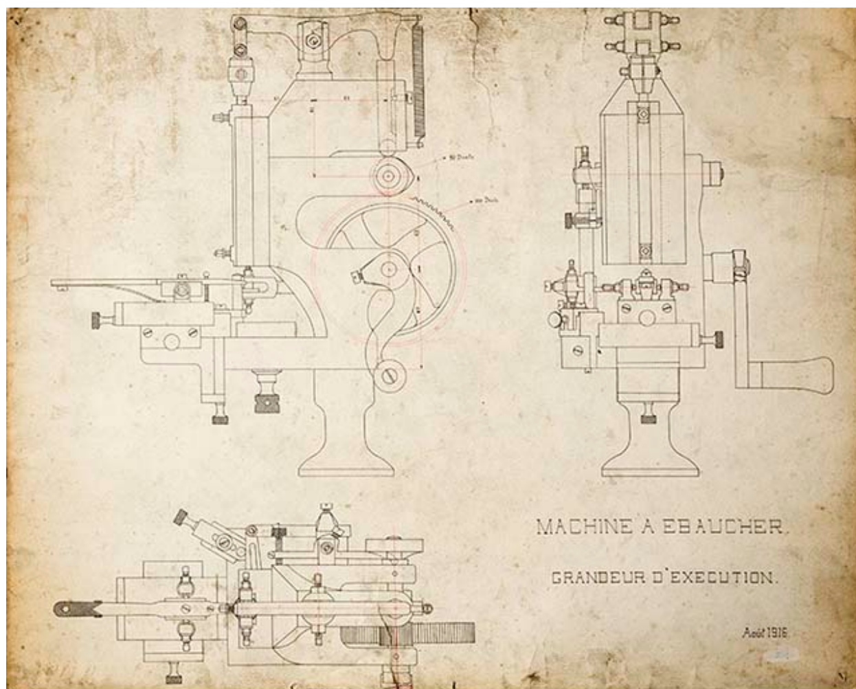
Machine à ébaucher. Grandeur d'exécution, août 1916.
