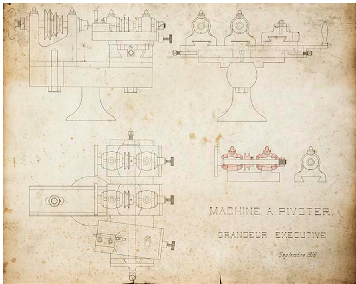
Machine à pivoter. Grandeur exécutive, septembre 1916.
