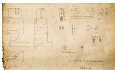
Machine à ébaucher. Détails, 1916. Phot. Yves Sancey, Autr. Adelin Berçot IVR43_20132501937NUC2A
