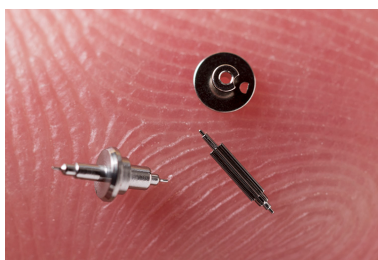
Exemples de composants fabriqués dans l'usine : axes de balancier, plateaux et pignons d'échappement.
