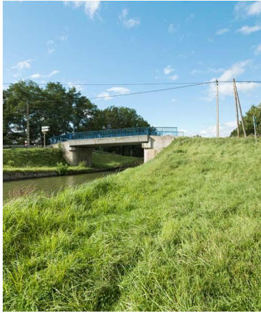
Vue d'ensemble du pont. Phot. Pierre-Marie Barbe-Richaud IVR26_20177100283NUC2A
