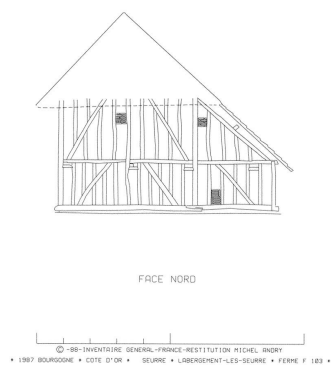
façade nord Dess. Alain Morelière, Dess. Michel Andry, Dess. A.P.A.I.G (Atelier de photogrammétrie architecturale de l'Inventaire général) IVR26_20122100815A2YY
