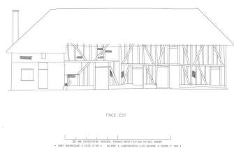
façade est Dess. Alain Morelière, Dess. Michel Andry, Dess. A.P.A.I.G (Atelier de photogrammétrie architecturale de l'Inventaire général) IVR26_20122100814A2YY
