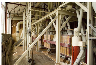
L'étage des plansichters. Phot. Jérôme Mongreville IVR43_20067000543NUCA
