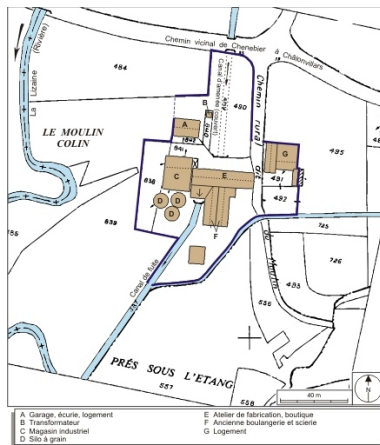
Plan-masse et de situation. Extrait du plan cadastral numérisé, 2008, section E, 1:1250. Source : Direction générale des Finances Publiques - Cadastre ; mise à jour : 2008. Dess. André Céréza IVR43_20087000153NUDA
