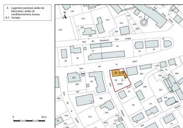
Plan-masse et de situation. Extrait du plan cadastral, 2015, section AI. Dess. Mathias Papigny IVR43_20152500643NUDA
