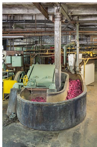
Usine à papier et cartonnerie dite manufacture de carton-cuir Hétier, Mesnay : pile raffineuse.
