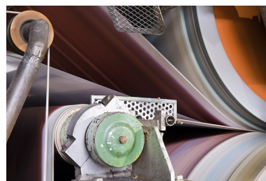
Usine de pâte à papier Paravicini-Maillard, actuellement Papeterie de Mandeure, Mandeure : passage de la feuille de papier entre les cylindres de pressage et d'égouttage.
