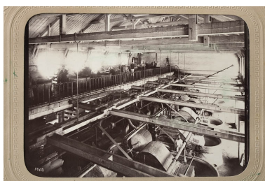
Usine de papeterie Outhenin-Chalandre et Fils, puis SA des Papeteries de France, Deluz : Atelier des piles raffineuses, [fin 19e ou début 20e siècle].
