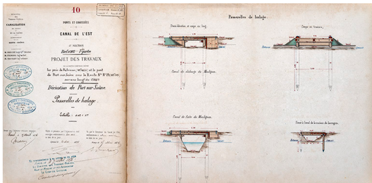
Canal de l'Est, projet des travaux - dérivation de Port-sur-Saône, passerelles de halage (1876).
