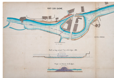
Profil en long suivant l'axe de la digue, à Port-sur-Saône [s.d]. Phot. Jérôme Mongreville, Phot. Service du canal de l'Est IVR43_20207000049NUC4A
