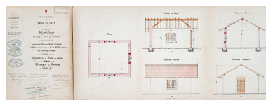
Canal de l'Est, projet des travaux - dérivation de Port-sur-Saône, magasin du barrage (1876). Phot. Jérôme Mongreville, Phot. Service du canal de l'Est IVR43_20207000035NUC4A
