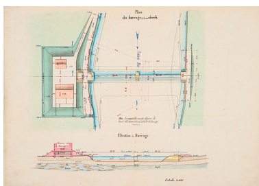
Canal de l'Est, projet des travaux de la dérivation de Port-sur-Saône - barrage mobile (1878) : détail du barrage et de ses abords. Phot. Jérôme Mongreville, Phot. Service du canal de l'Est IVR43_20207000034NUC4A
