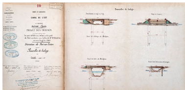
Canal de l'Est, projet des travaux - dérivation de Port-sur-Saône, passerelles de halage (1876). Phot. Jérôme Mongreville, Phot. Service du canal de l'Est IVR43_20207000036NUC4A
