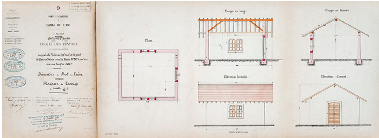
Canal de l'Est, projet des travaux - dérivation de Port-sur-Saône, magasin du barrage (1876).
