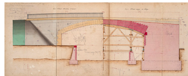
Amélioration du cours de la Saône entre Port-sur-Saône, construction de la dérivation de Port-sur-Saône - pont sur la dérivation (1876) : demi-coupe. Phot. Jérôme Mongreville, Phot. Service du canal de l'Est IVR43_20207000052NUC4A
