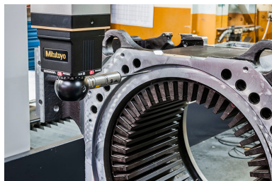
Machine de contrôle tridimensionnel. Phot. Jérôme Mongreville IVR43_20162500177NUC4A
