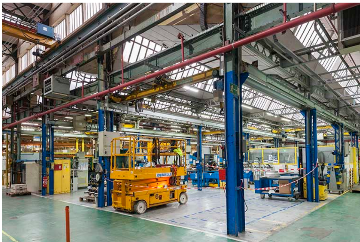
Ossature et charpente métallique de l'atelier central.
