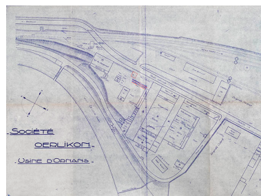
Plan de l'usine d'Ornans, tirage, 1939.
