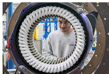
Atelier de bobinage. Montage des barres de cuivre sur un stator. Phot. Jérôme Mongreville IVR43_20162500160NUC4A
