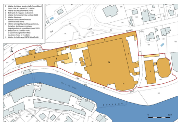
Plan-masse et de situation. Extrait du plan cadastral, 2016, section AS.
