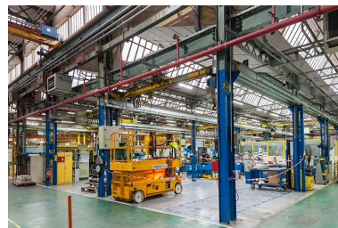
Ossature et charpente métallique de l'atelier central. Phot. Jérôme Mongreville IVR43_20162500150NUC4A
