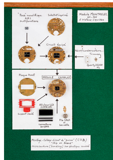
Composants d'un module à quartz Montrelec 61-NU à cristaux liquides, étudié par le Cetehor (1976). (Collection Cetehor, Besançon). Phot. Sonia Dourlot IVR43_20192500308NUC4A
