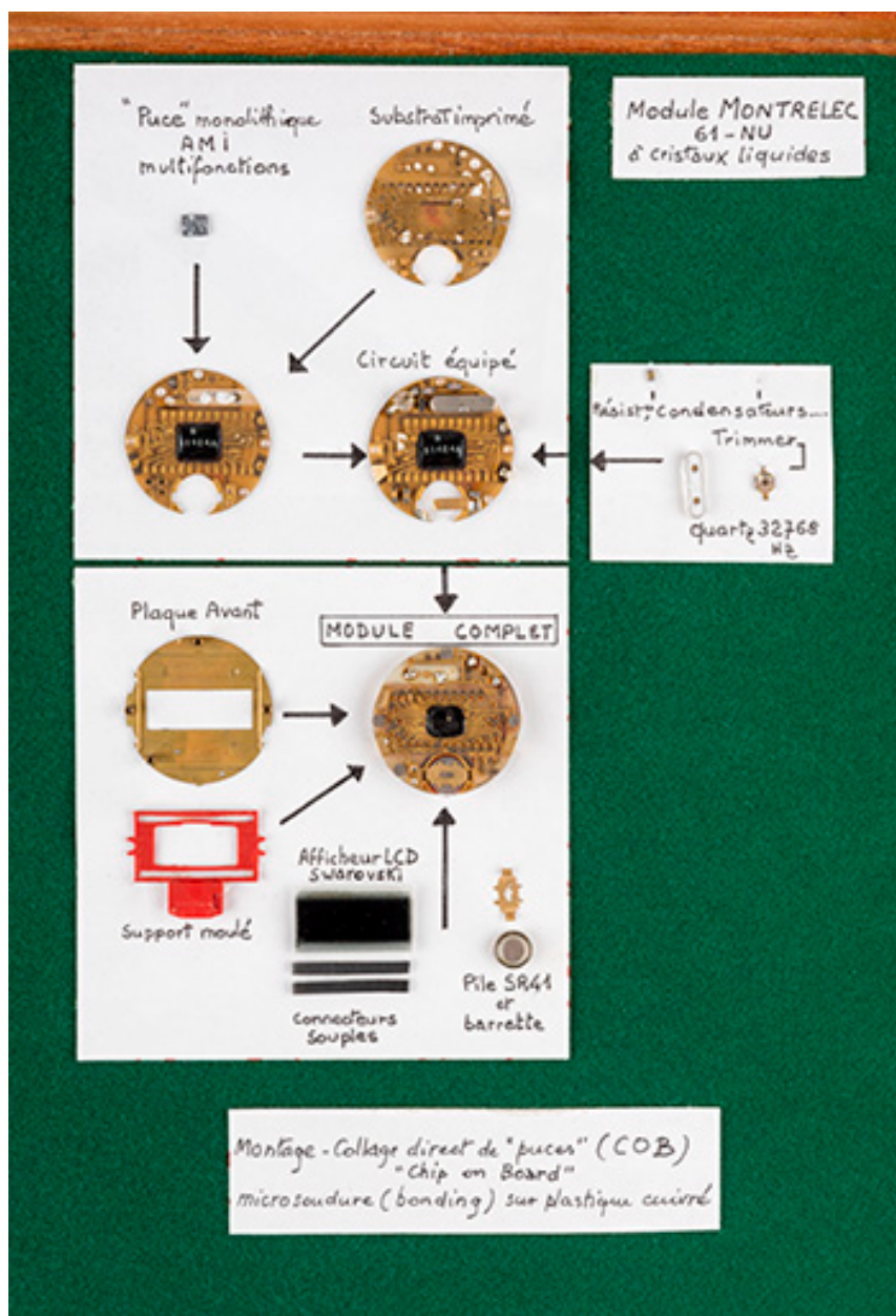
Composants d'un module à quartz Montrelec 61-NU à cristaux liquides, étudié par le Cete hor (1976). (Collection Cete hor, Besançon).
