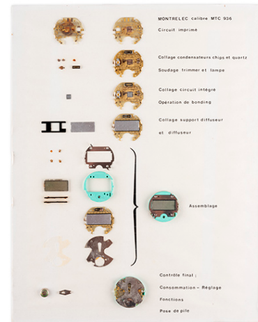
Composants et phases de montage d'un module à quartz Montrelec MTC 936, étudié par le Cetehor. (Collection Cetehor, Besançon). Phot. Sonia Dourlot IVR43_20192500299NUC4A
