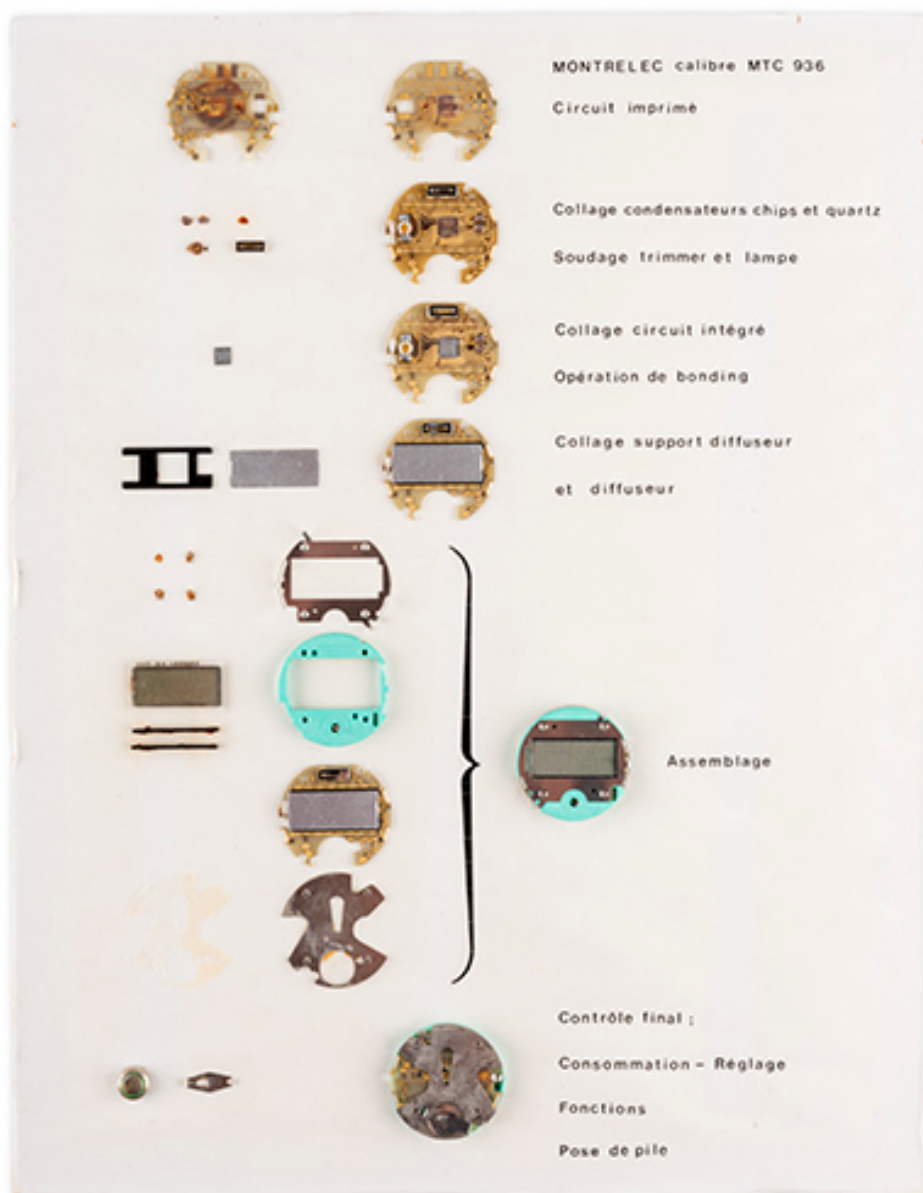
Composants et phases de montage d'un module à quartz Montrelec MTC 936, étudié par le Cetehor. (Collection Cetehor, Besançon).
