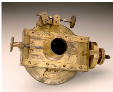
Le micromètre, vu de face. Phot. Jérôme Mongreville IVR43_20032500756XA
