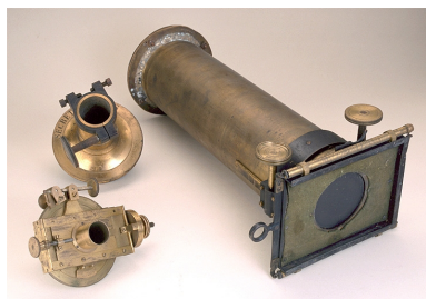
Vue d'ensemble du tube avec porte-plaque à crémaillère (à droite), accompagné du micromètre (au 1er plan) et du porte-oculaire (au 2e plan). Phot. Jérôme Mongreville IVR43_20032500752XA
