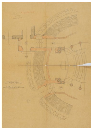
Théâtre [détail des accès]. 31 juillet 1906. Phot. Pierre-Marie Barbe- Richaud, Autr. Ernest Sanson IVR26_20257100314NUC4A
