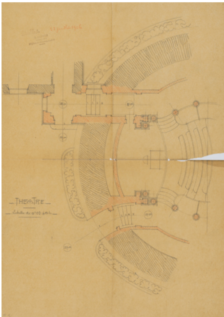
Théâtre [détail des accès]. 31 juillet 1906.
