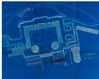
La Verrerie [plan-masse et de situation]. S.d. [1905]. Phot. Pierre-Marie Barbe- Richaud, Autr. auteur inconnu IVR26_20257100325NUC2A
