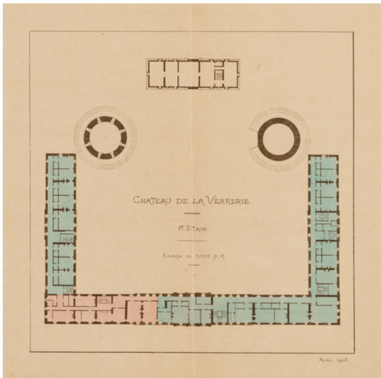
Château de la Verrerie. 1er étage. Avril 1905.
