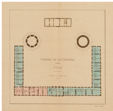
Château de la Verrerie. 1er étage. Avril 1905. Phot. Pierre-Marie Barbe- Richaud, Autr. Landrevault IVR26_20257100309NUC2A
