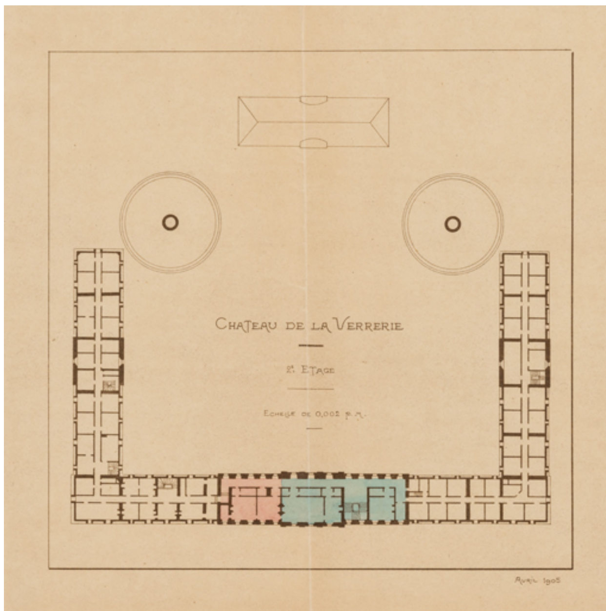
Château de la Verrerie. 2e étage. Avril 1905.
