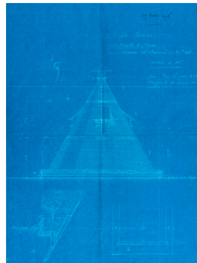
La Verrerie. Chapelle et Théâtre. Lucarnes et jardinières. 29 mars 1906. Phot. Pierre-Marie Barbe- Richaud, Autr. auteur inconnu
