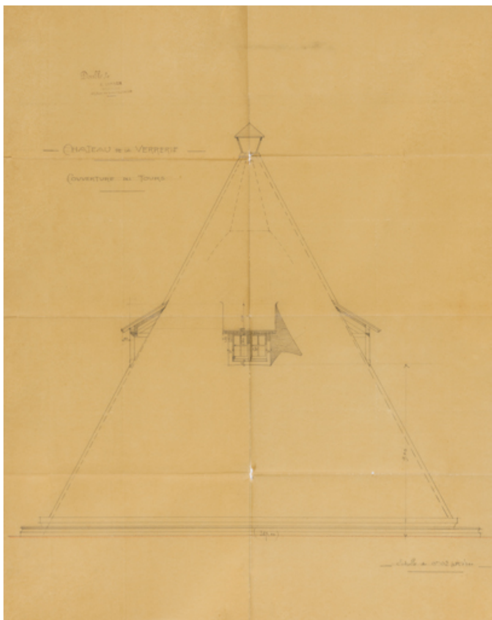
Château de la Verrerie. Couverture des tours. S.d. [1906 ?].
