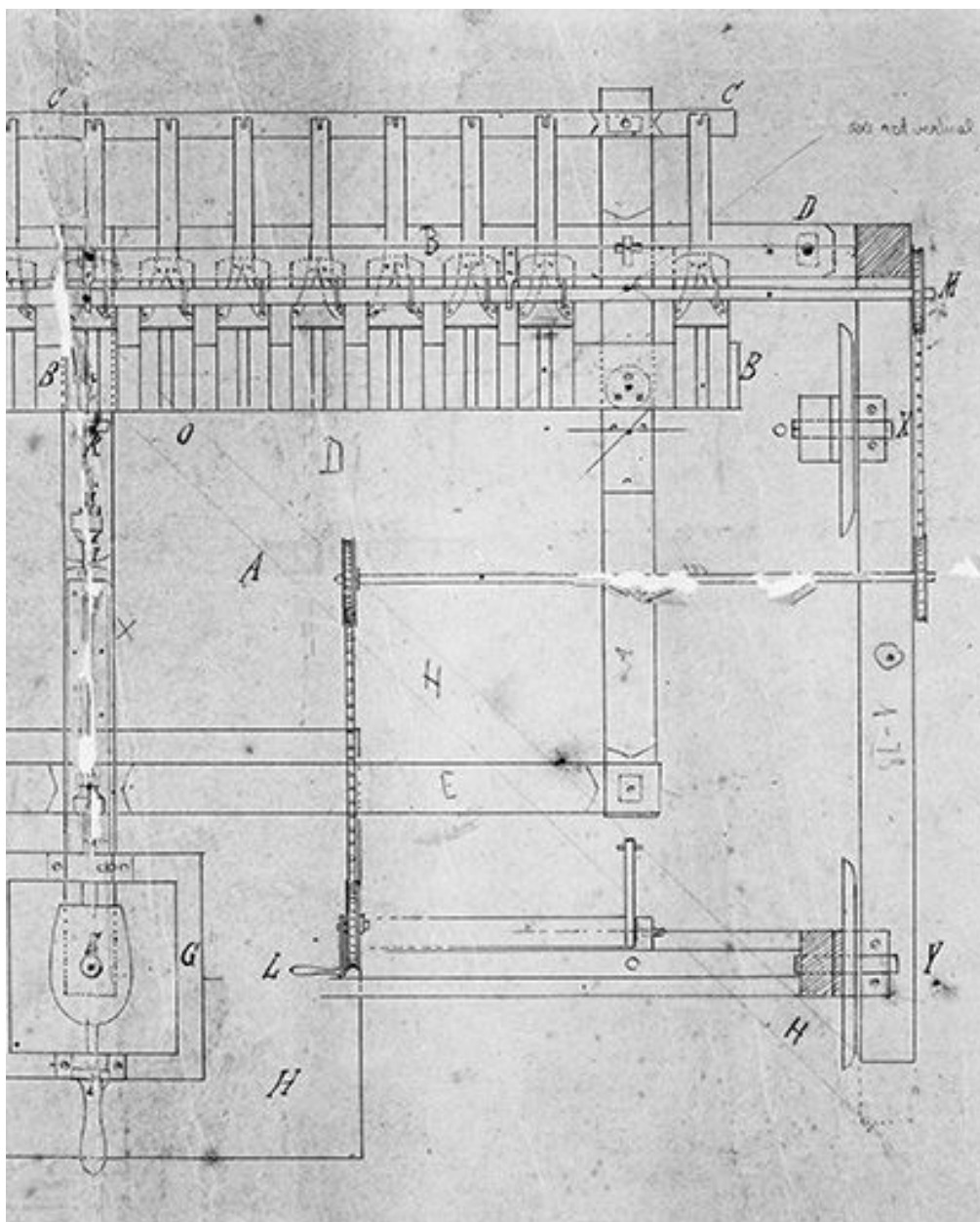
Plan de la machine : détail de la partie droite du plan.
