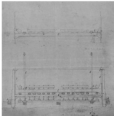
Elévation partielle de la face postérieure donnant les dessins du système d'entraînement des fraises et de fixation des ébauchons, et d'une partie du bâti mobile. Phot. Jérôme Mongreville IVR43_20003901207V
