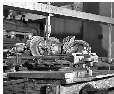
Modèle (d'Artagnan) et son support mobile, vus de trois quarts avant gauche. Manœuvré à l'aide des poignées, le support glisse sur une plaque métallique, chaque détail du modèle pouvant ainsi être retransmis par le palpeur vertical. Phot. Jérôme Mongreville IVR43_20003901200X
