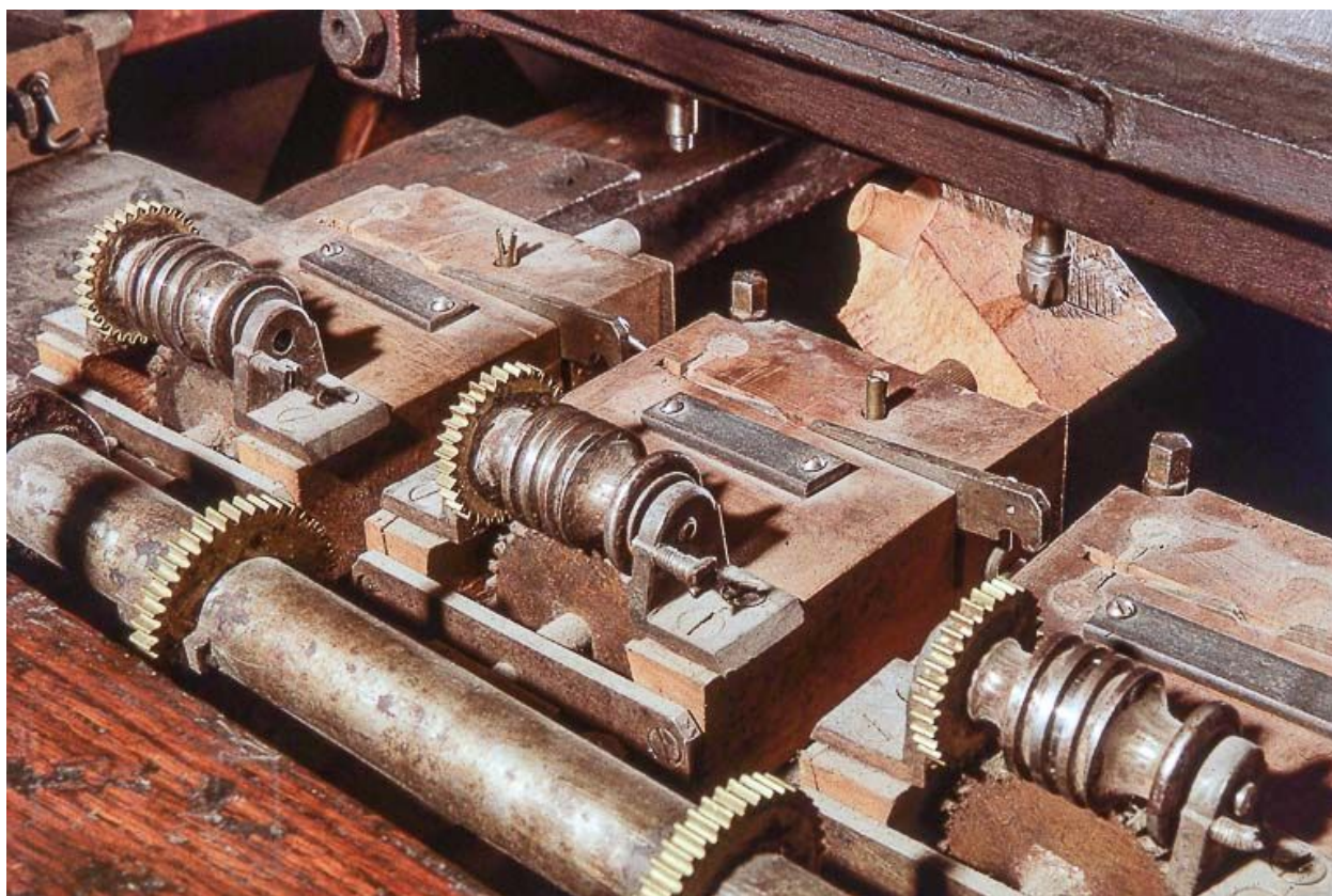
Face arrière : engrenages permettant la rotation simultanée des ébauchons.
