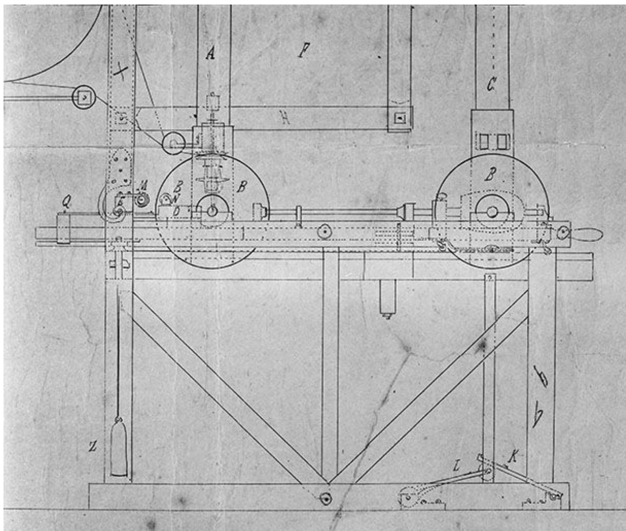
Elévation de la face latérale gauche : détail de la partie centrale du plan.
