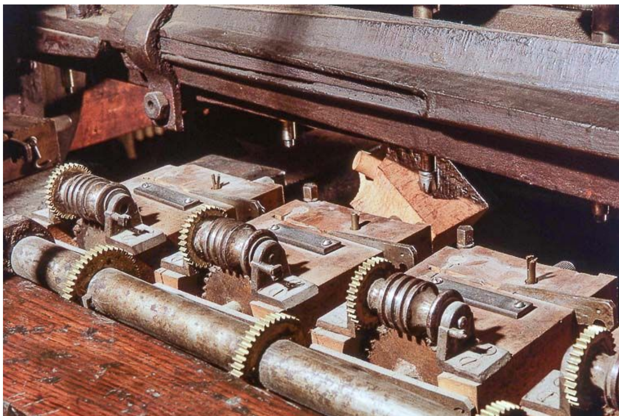
Face arrière : engrenages permettant la rotation simultanée des ébauchons (vue rapprochée).
