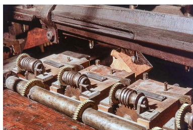
Face arrière : engrenages permettant la rotation simultanée des ébauchons (vue rapprochée). Phot. Jérôme Mongreville IVR43_20003901192ZA
