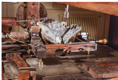
Modèle (d'Artagnan) et son support mobile, vus de trois quarts arrière gauche. Manœuvré à l'aide de poignées, le support glisse sur une plaque métallique, chaque détail du modèle pouvant ainsi être retransmis par le palpeur vertical. Phot. Jérôme Mongreville IVR43_20003901199ZA
