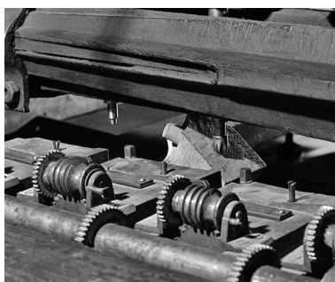
Face arrière : engrenages permettant la rotation simultanée des ébauchons (vue rapprochée). Phot. Jérôme Mongreville IVR43_20003901191X
