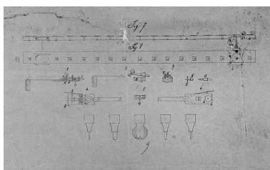
Dessins de détails : éléments du bâti, engrenages, système de rotation des supports d'ébauchons, fraises. Phot. Jérôme Mongreville IVR43_20003901206V
