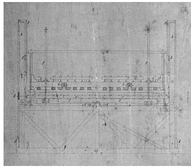
Elévation de la face postérieure. Phot. Jérôme Mongreville IVR43_20003901204V
