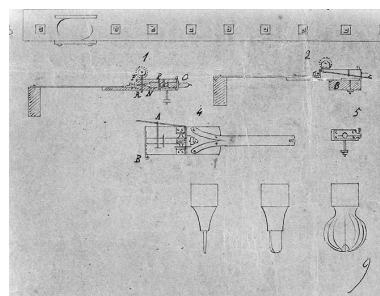
Dessins de détails [partie droite du plan] : éléments du bâti, engrenages, système de rotation des supports d'ébauchons, fraises. Phot. Jérôme Mongreville IVR43_20003901153X
