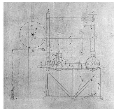
Elévation de la face latérale gauche. Phot. Jérôme Mongreville IVR43_20003901203V
