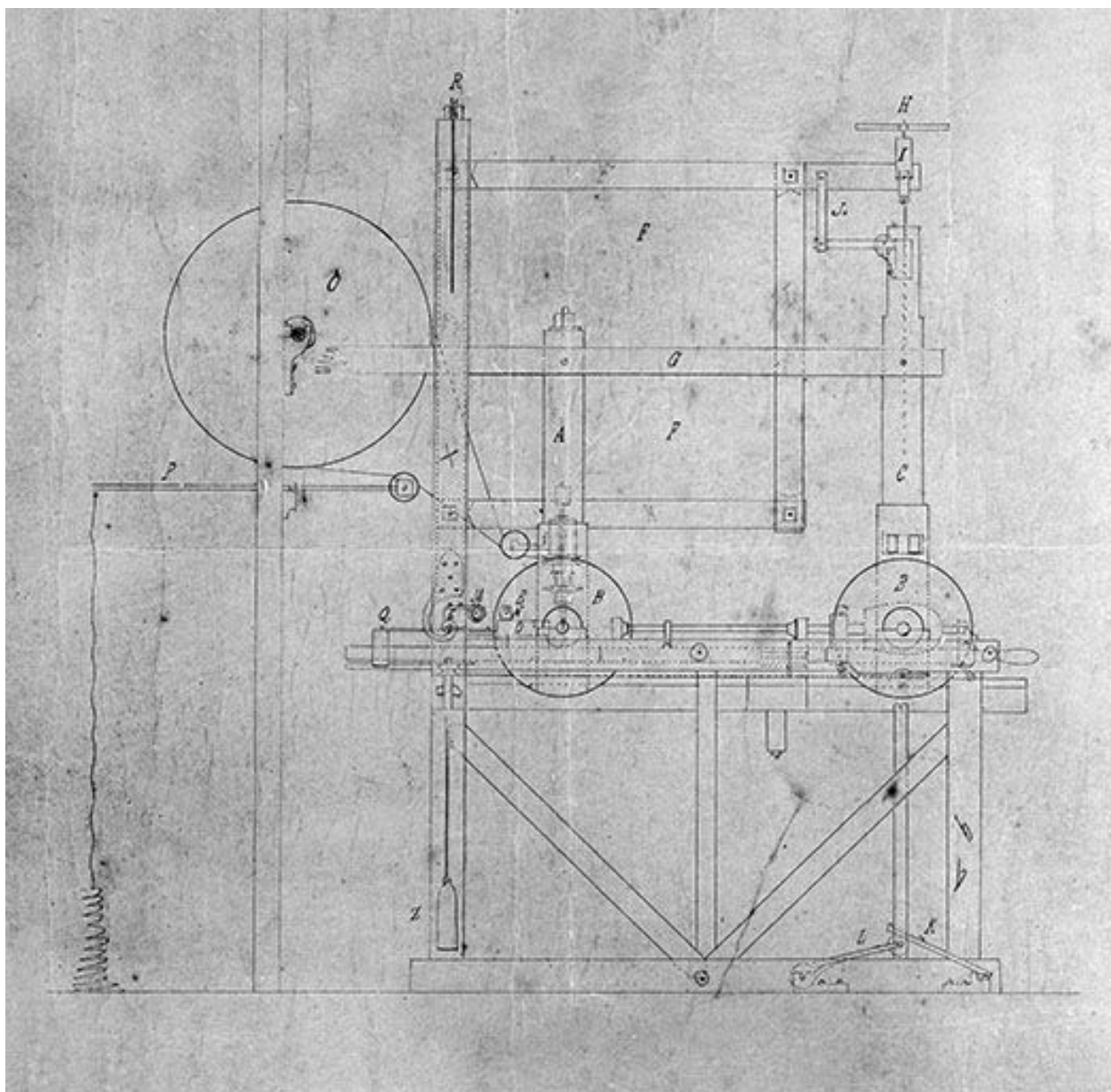
Elévation de la face latérale gauche.
