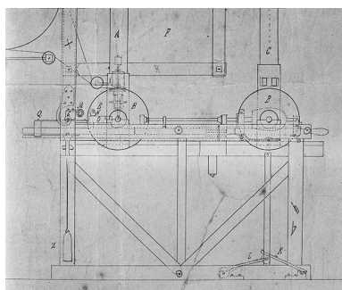
Elévation de la face latérale gauche : détail de la partie centrale du plan. Phot. Jérôme Mongreville IVR43_20003901149X
