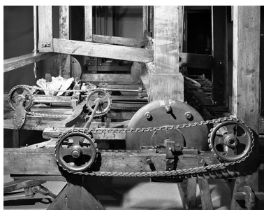
Face latérale droite. Aux premier et second plans, système de renvoi par chaîne permettant la rotation simultanée du modèle et des ébauchons. Phot. Jérôme Mongreville IVR43_20003901209V
