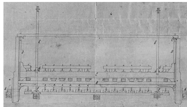
Elévation partielle de la face postérieure : détail du plan montrant le système d'entraînement des fraises et de fixation des ébauchons. Phot. Jérôme Mongreville IVR43_20003901150X
