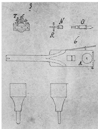
Dessins de détails [partie gauche du plan] : engrenages, système de rotation des supports d'ébauchons, fraises. Phot. Jérôme Mongreville IVR43_20003901151X
