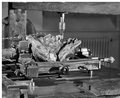
Modèle (d'Artagnan) et son support mobile, vus de trois quarts arrière gauche. Manœuvré à l'aide de poignées, le support glisse sur une plaque métallique, chaque détail du modèle pouvant ainsi être retransmis par le palpeur vertical. Phot. Jérôme Mongreville IVR43_20003901198X
