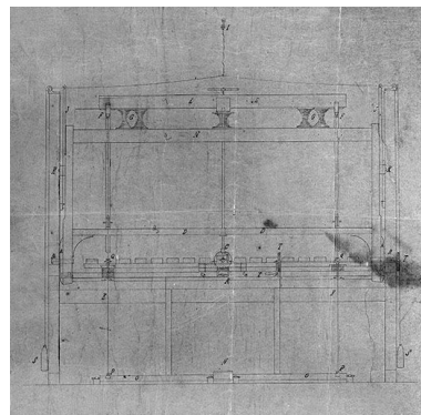
Elévation de la face antérieure. Phot. Jérôme Mongreville IVR43_20003901208V
