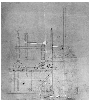
Elévation de la face latérale droite. Phot. Jérôme Mongreville IVR43_20003901202V
