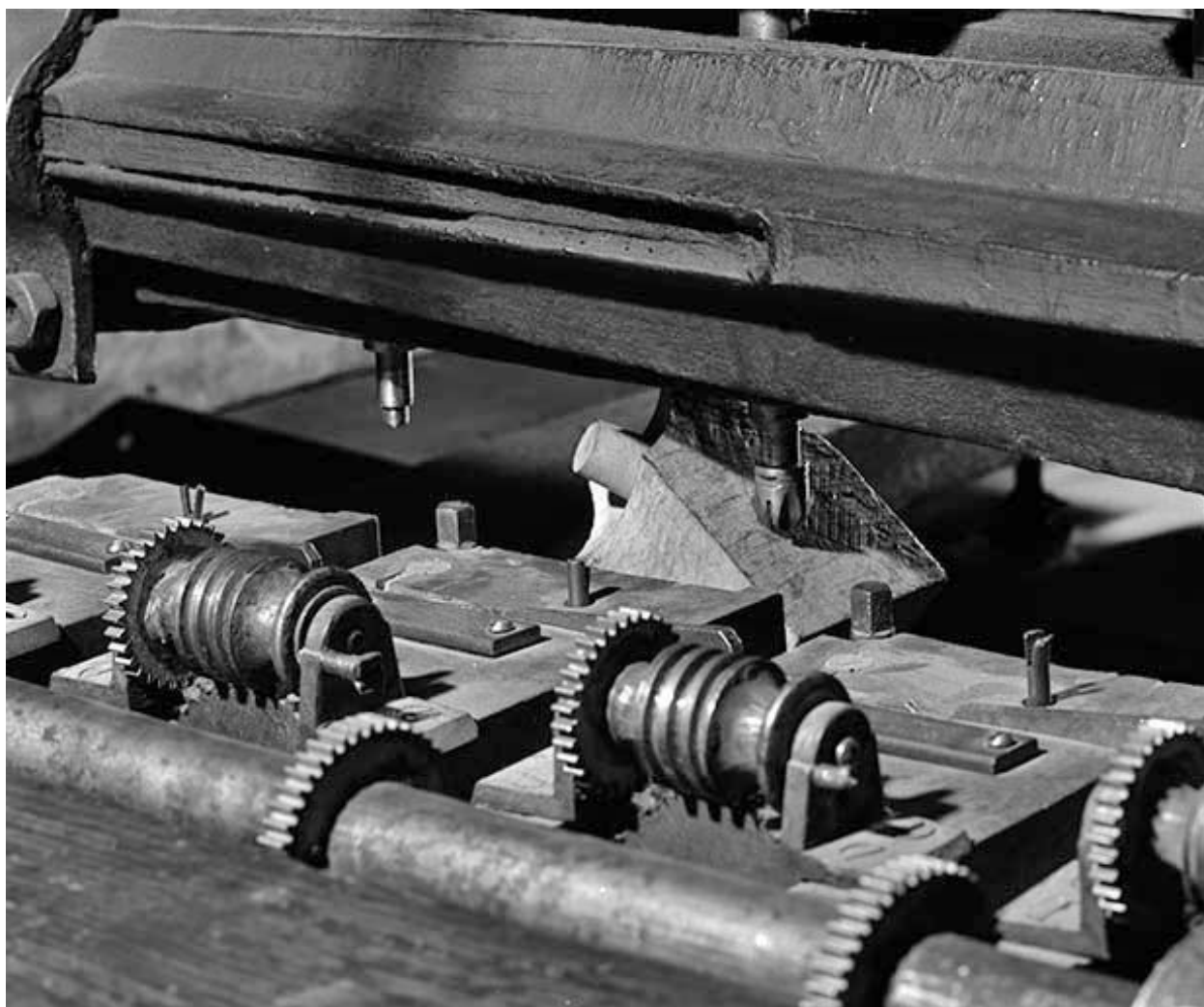
Face arrière : engrenages permettant la rotation simultanée des ébauchons (vue rapprochée).
