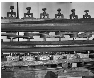
Face arrière : système moteur des fraises et supports des ébauchons. Le mouvement est transmis aux fraises à l'aide des poulies et des courroies en partie supérieure. Les ébauchons sont emboîtés dans les mandrins coniques en partie basse. Phot. Jérôme Mongreville IVR43_20003901197X
