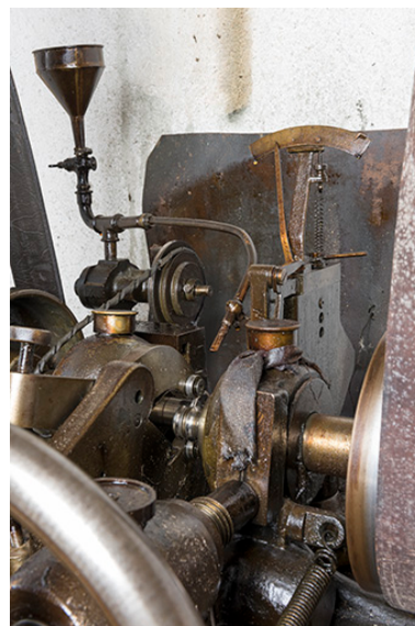
Partie travaillante (sous le tuyau d'amenée d'huile). Phot. Sonia Dourlot IVR43_20182501130NUC4A
