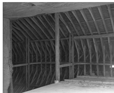
Charpente vue depuis la porte d'entrée du narthex. Phot. Michel Thierry IVR26_19748900764X
