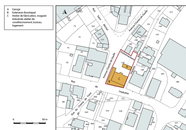
Plan-masse et de situation. Extrait du plan cadastral, 2017, section AF, 1/1 000. Dess. Bertrand Turina IVR43_20182501353NUDA
