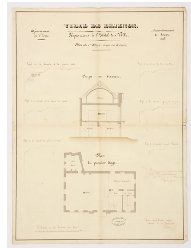
Ville de Brienon. Réparations à l'hôtel de ville. Plan du 1er étage, coupe en travers. 29 janvier 1848.
