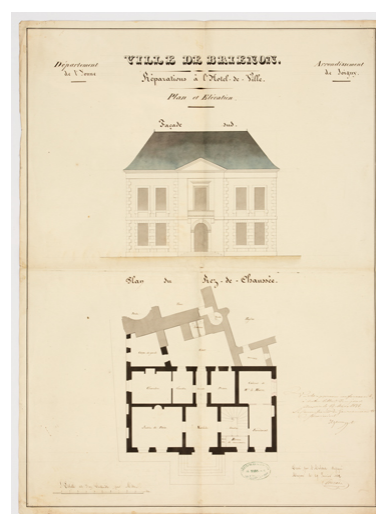
Ville de Brienon. Réparations à l'hôtel de ville. Plan et élévation. 29 janvier 1848. Phot. Pierre-Marie Barbe-Richaud, Autr. Philippe Pourain IVR26_20238900503NUC4A
