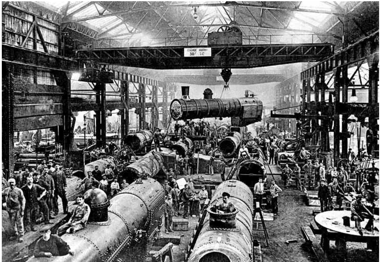
Montage des chaudières de locomotives.
