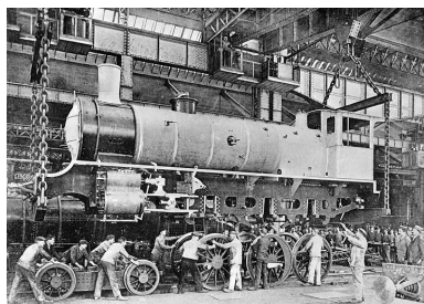
Montage d'une locomotive. Phot. Jérôme Mongreville IVR43_20019000084X
