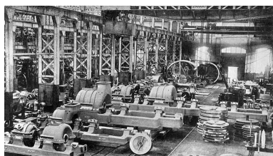
Atelier des turbines à vapeur. Phot. Jérôme Mongreville IVR43_20019000086X
