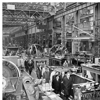
Hall du gros matériel électrique. Phot. Jérôme Mongreville IVR43_20029000198X
