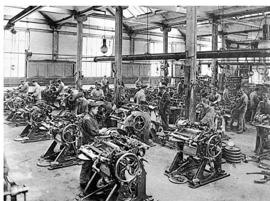
Montage des peigneuses. Phot. Jérôme Mongreville, Autr. Ernest (photographe) Mésière IVR43_20019000187X
