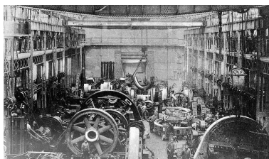
Intérieur d'atelier de la Société Alsacienne. Phot. Jérôme Mongreville IVR43_20019000173X
