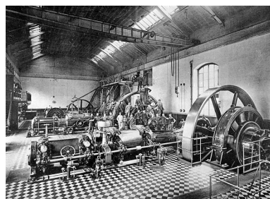
Station centrale d'électricité. Phot. Jérôme Mongreville, Autr. Ernest (photographe) Mésière IVR43_20019000224X
