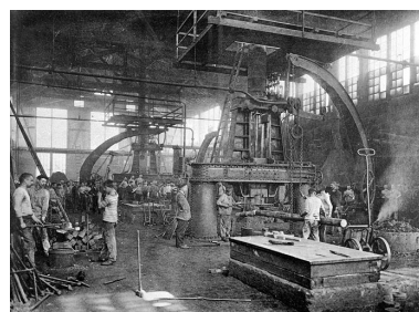
Forge - Marteaux-pilons de 2000 kgs double effet. Phot. Jérôme Mongreville, Autr. Ernest (photographe) Mésière IVR43_20019000134X
