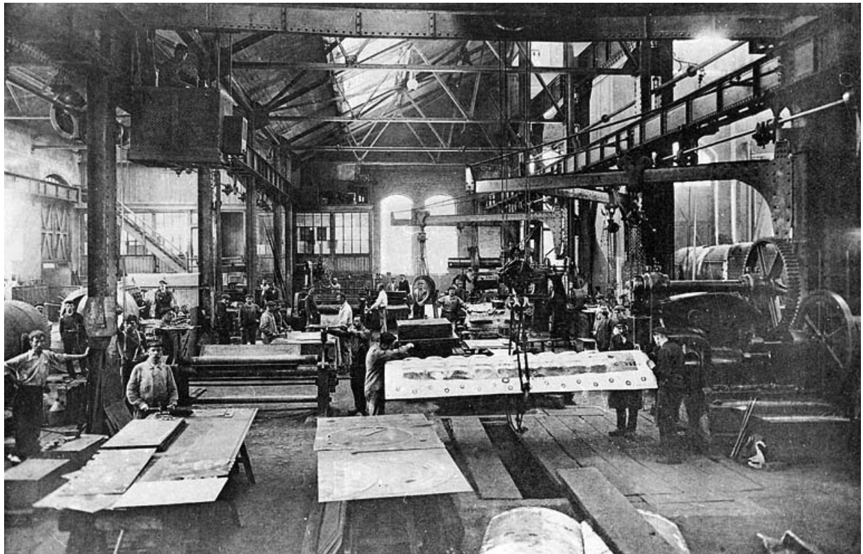
Chaudronnerie - Cintrage des tôles.
