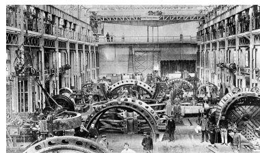
Belfort industriel. Atelier des dynamos. Phot. Jérôme Mongreville IVR43_20019000112X
