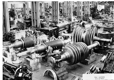
Hall de montage des rotors pour turbines à vapeur. Phot. Jérôme Mongreville, Autr. auteur inconnu IVR43_20029000191X
