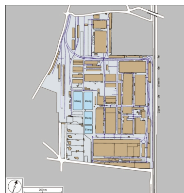
Plan-masse en 1933. D'après un plan de l'usine, janvier 1933, mis au net par A. Céréza, échelle 1:5500. Dess. André Céréza IVR43_20039000088NUDA
