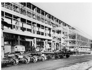
Construction des ateliers et bureaux du gros matériel électrique tournant. Phot. Jérôme Mongreville IVR43_20029000209X
