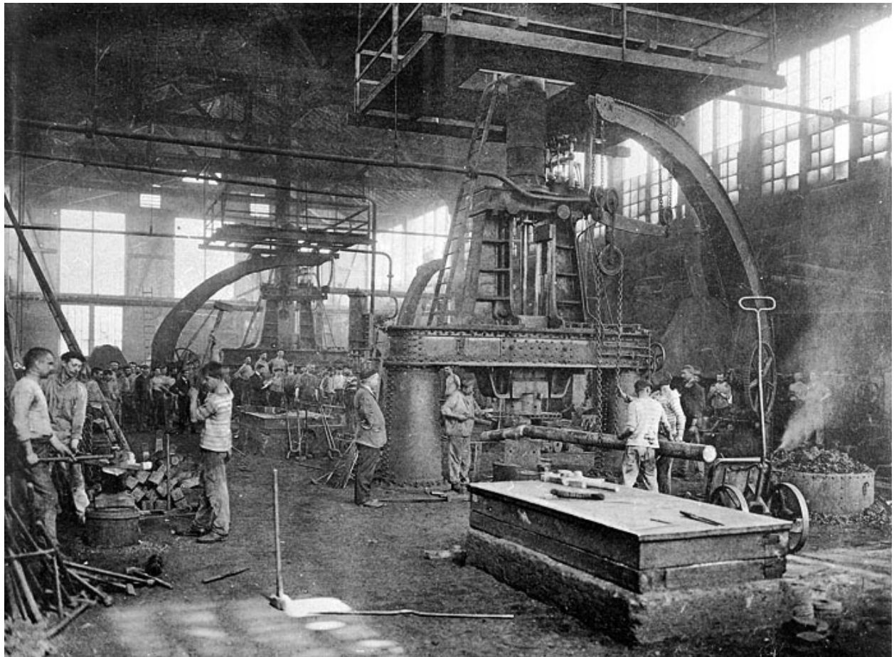
Forge - Marteaux-pilons de 2000 kgs double effet.
