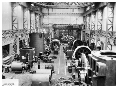
Hall des grandes dynamos. Phot. Jérôme Mongreville IVR43_20019000171X
