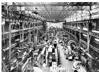
Atelier des grandes dynamos. Phot. Jérôme Mongreville IVR43_20019000118X
