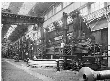
Hall de gros usinage : tour à usiner des pièces de 8 m de diamètre, 4 m de haut et 110 t. Phot. Jérôme Mongreville IVR43_20029000190X
