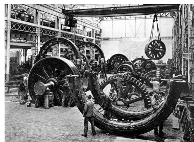
Atelier des grandes dynamos - Finissage des machines. Phot. Jérôme Mongreville, Autr. Ernest (photographe) Mésière IVR43_20019000221X
