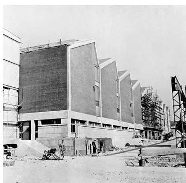
Construction de l'atelier d'usinage Traction. Phot. Jérôme Mongreville IVR43_20029000208X
