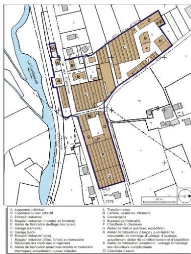
Plan-masse et de situation. Extrait du plan cadastral numérisé, 2008, section B, 1:1000 réduit à 1:2000. Source : Direction générale des Finances Publiques - Cadastre ; mise à jour : 2008. Dess. André Céréza IVR43_20087000250NUDA
