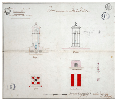
Plan pour la construction d'une fontaine publique. 1841. Repro. Jérôme Mongreville, Autr. Charles Alexandre Ringuelet IVR43_20197000026NUC4A
