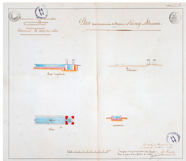
Plan pour la construction de bassins de puisage et d'abreuvoir. 1841. Repro. Jérôme Mongreville, Autr. Charles Alexandre Ringuelet IVR43_20197000025NUC4A
