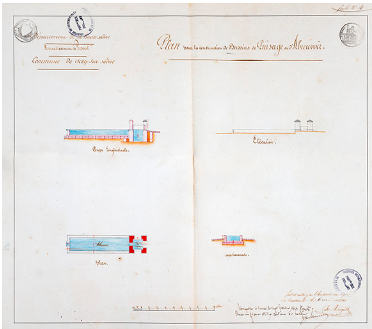
Plan pour la construction de bassins de puisage et d'abreuvoir. 1841.
