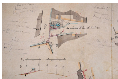
Plan de construction de rigoles pavées autour de la fontaine de la Croix de Pierre à Sceaux-sur-Saône-et-Saint-Albin, détail. [1866]. Repro. Jérôme Mongreville, Phot. auteur inconnu IVR43_20197000035NUC4A
