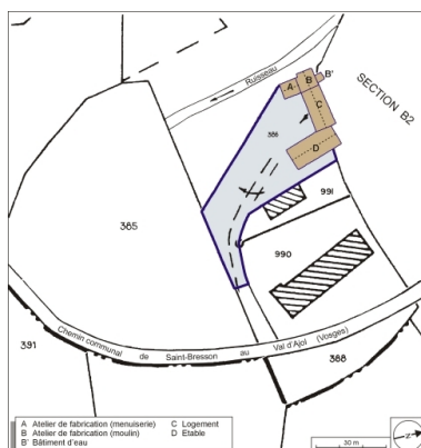
Plan-masse et de situation. Extrait du plan cadastral numérisé, 2005, section B, 1:2500 agrandi à 1:1000. Dess. André Céréza IVR43_20067000003NUDA
