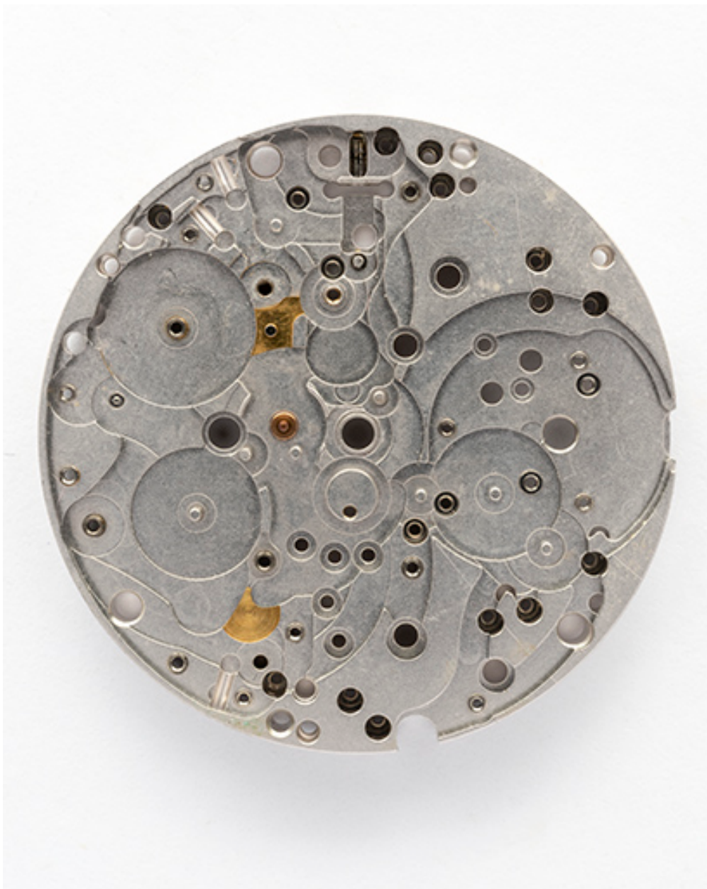
Platine, face côté cadran.
