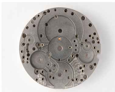
Platine, face côté fond. Phot. Sonia Dourlot IVR43_20182501208NUC4A
