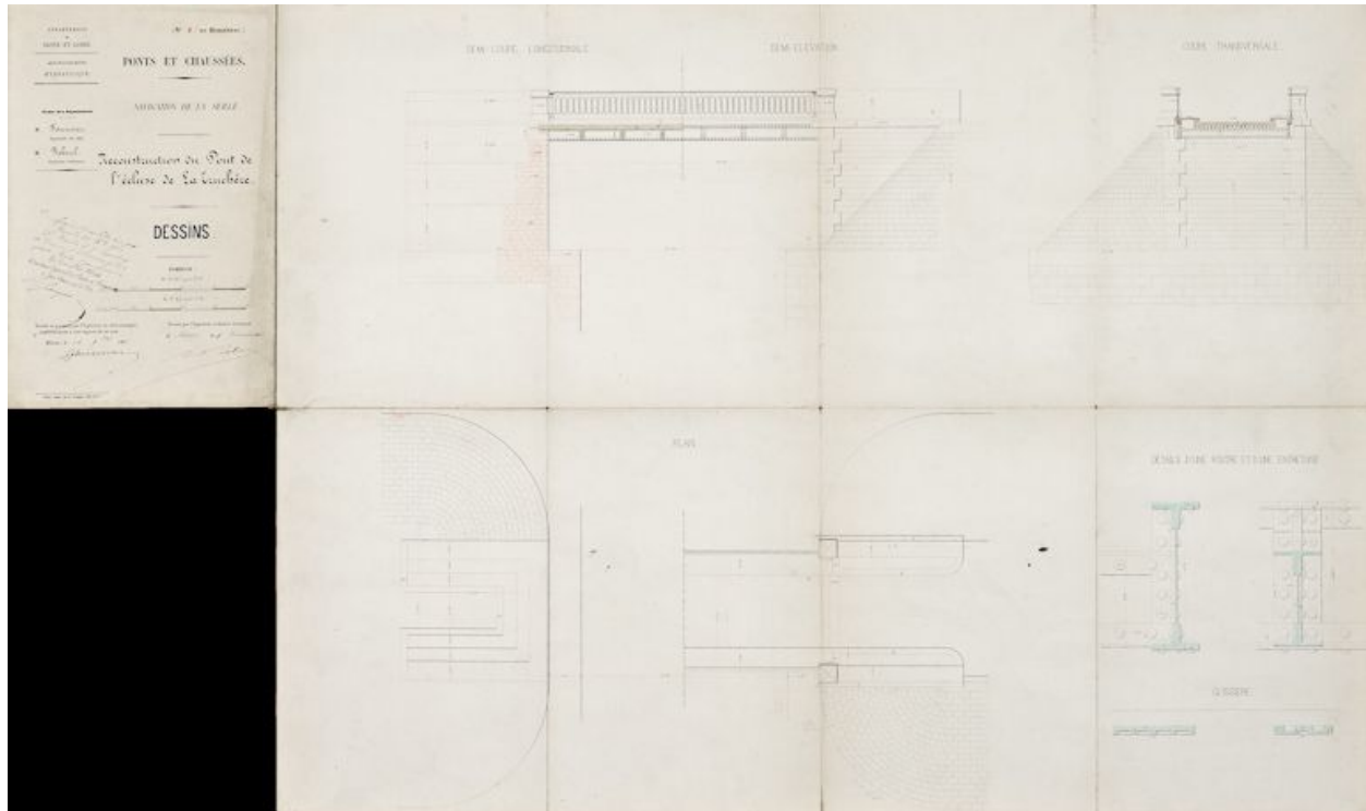
"Reconstruction du pont de l'écluse de La Truchère : Dessins". (Archives VNF-direction territoriale Centre-Bourgogne ; subdivision de Montceau-les-Mines)
