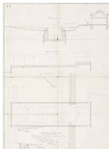
Projet d'exhaussement de l'écluse de la Truchère, du perfectionnement de ses abords et du rattachement de cet ouvrage au barrage", par l'ingénieur Delarue, le 20 décembre 1824. Coupe du sas et de la maison éclésièr. (Archives VNF-direction territoriale Centre-Bourgogne ; subdivision de Montceau-les-Mines) Phot. Jean-Luc Duthu, Autr. Delarue IVR26_20120100016NUC2A
