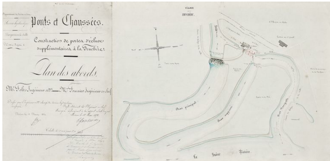
"Construction de portes d'écluse supplémentaires à La Truchère, plan des abords". 1854 (Archives VNF-direction territoriale Centre-Bourgogne ; subdivision de Montceau-les-Mines)
