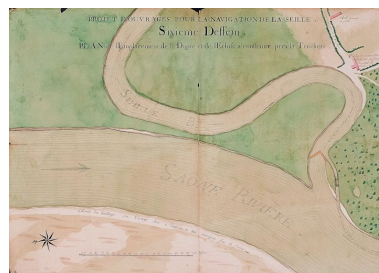
"Projet d'ouvrages pour la navigation de la Seille. Sixième dessin. Plan de l'emplacement de la digue et de l'écluse à construire près la Truchère". Il s'agit probablement d'un plan d'avant 1784. (Archives VNF-direction territoriale Centre-Bourgogne ; subdivision de Montceau-les-Mines) Phot. Jean-Luc Duthu IVR26_20120100010NUC2A
