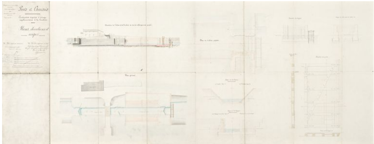
Plans, élévations et coupes du site de l'écluse de La Truchère. 1854 (Archives VNF-direction territoriale Centre-Bourgogne ; subdivision de Montceau-les-Mines)
