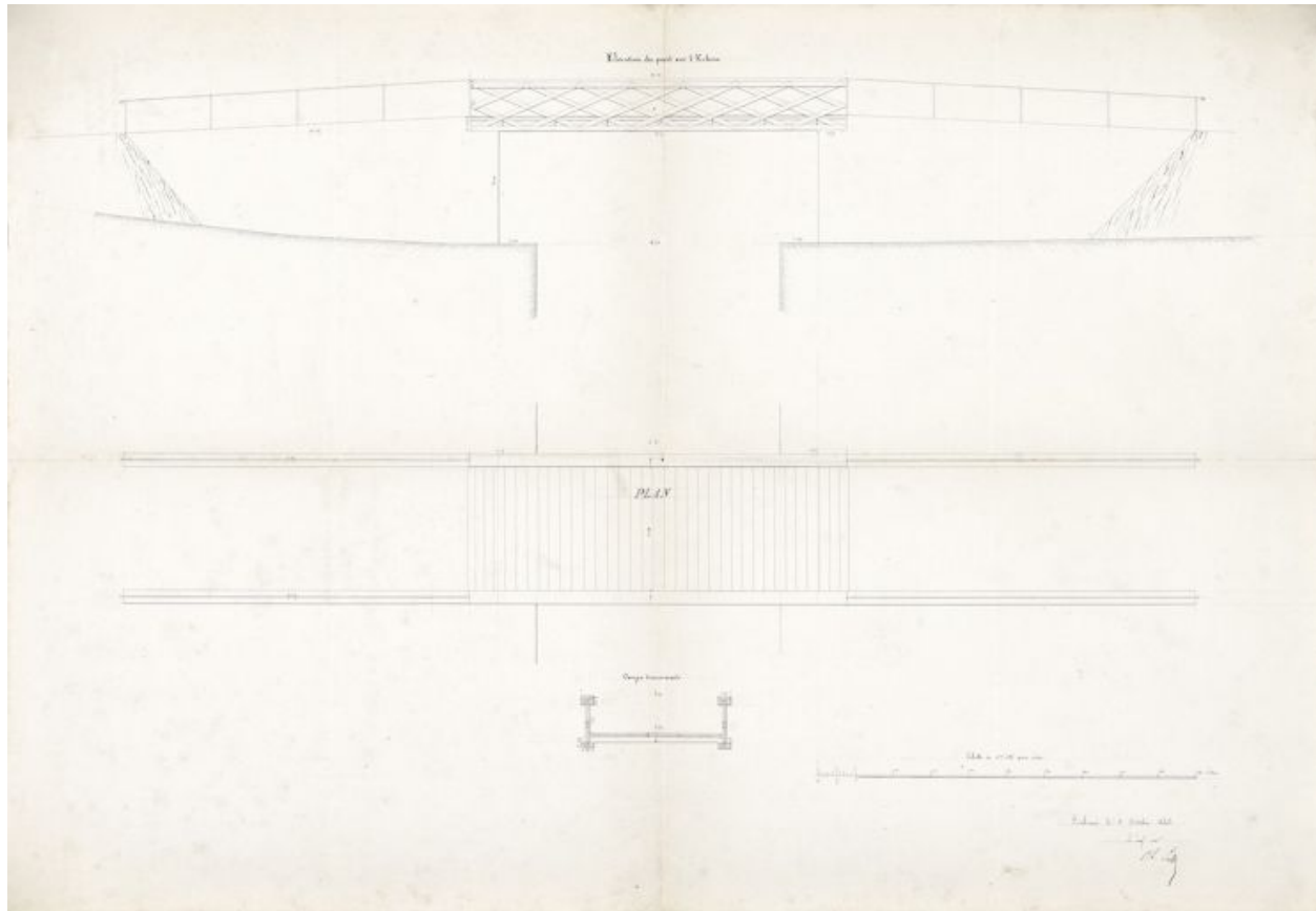
Plan du pont en charpente à construire sur l'écluse de La Truchère. Plan, coupe et élévation. 1846. (Archives VNF-direction territoriale Centre-Bourgogne ; subdivision de Montceau-les-Mines)
