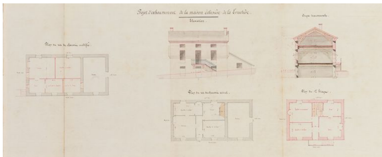
"Projet d'exhaussement des ponts. Plans - Profils - Elevations - Coupes" : détail du projet d'exhaussement de la maison éclusière de la Truchère. 1855. (VNF-direction territoriale Centre-Bourgogne ; subdivision de Montceau-les-Mines)
