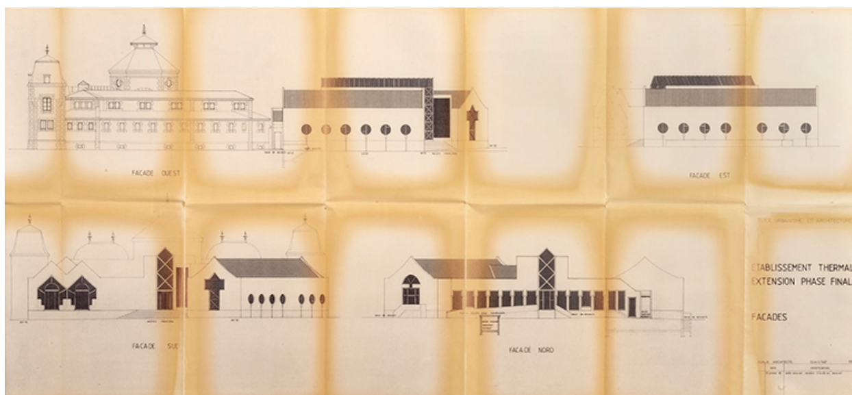
Façades, projet (décembre 1981).
