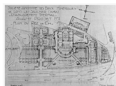
Plan, projet de transformation et d'agrandissement (1925). Phot. Yves Sancey, Autr. Fernand Grizet IVR43_19833900710V
