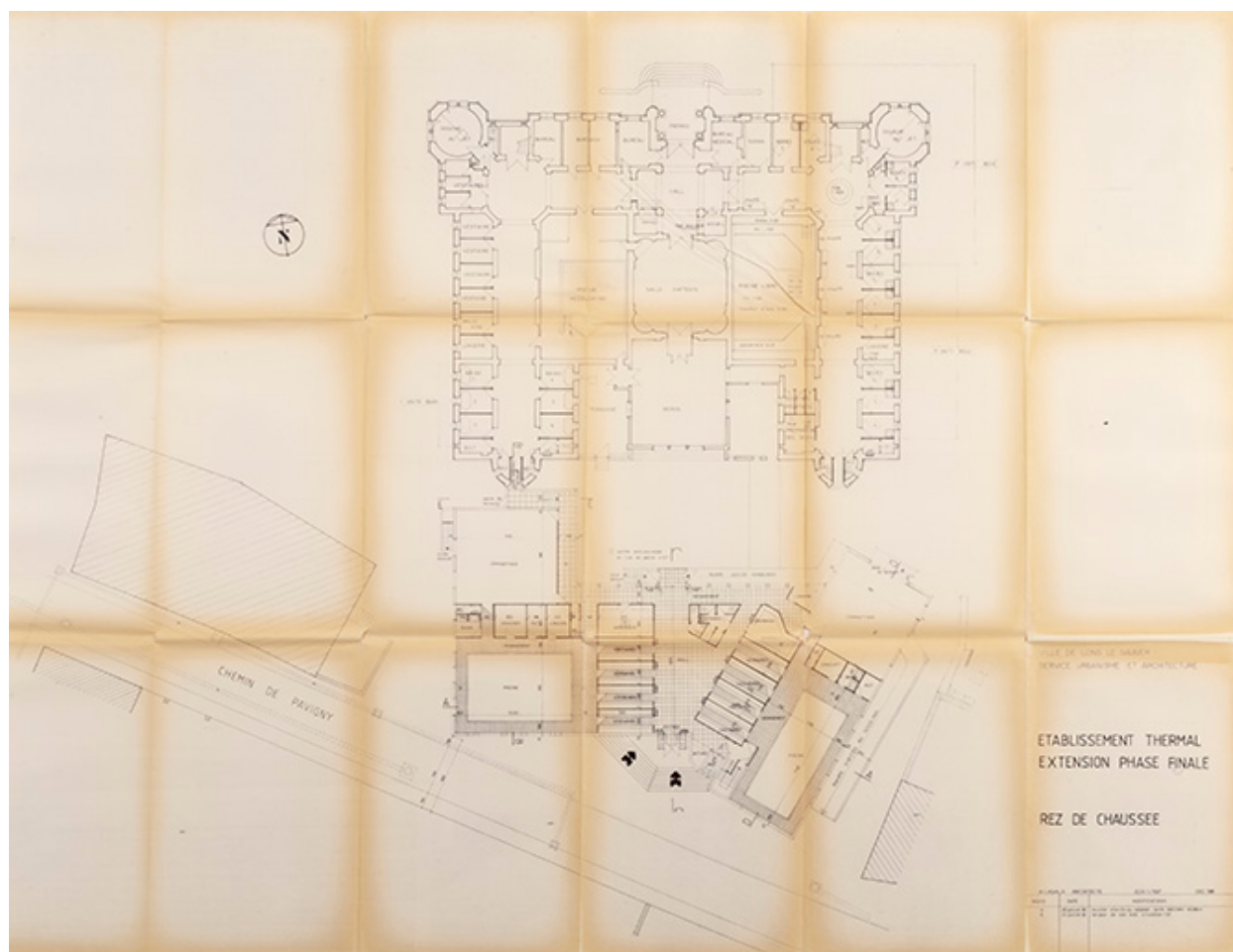
Plan du rez-de-chaussée, projet (décembre 1981).
