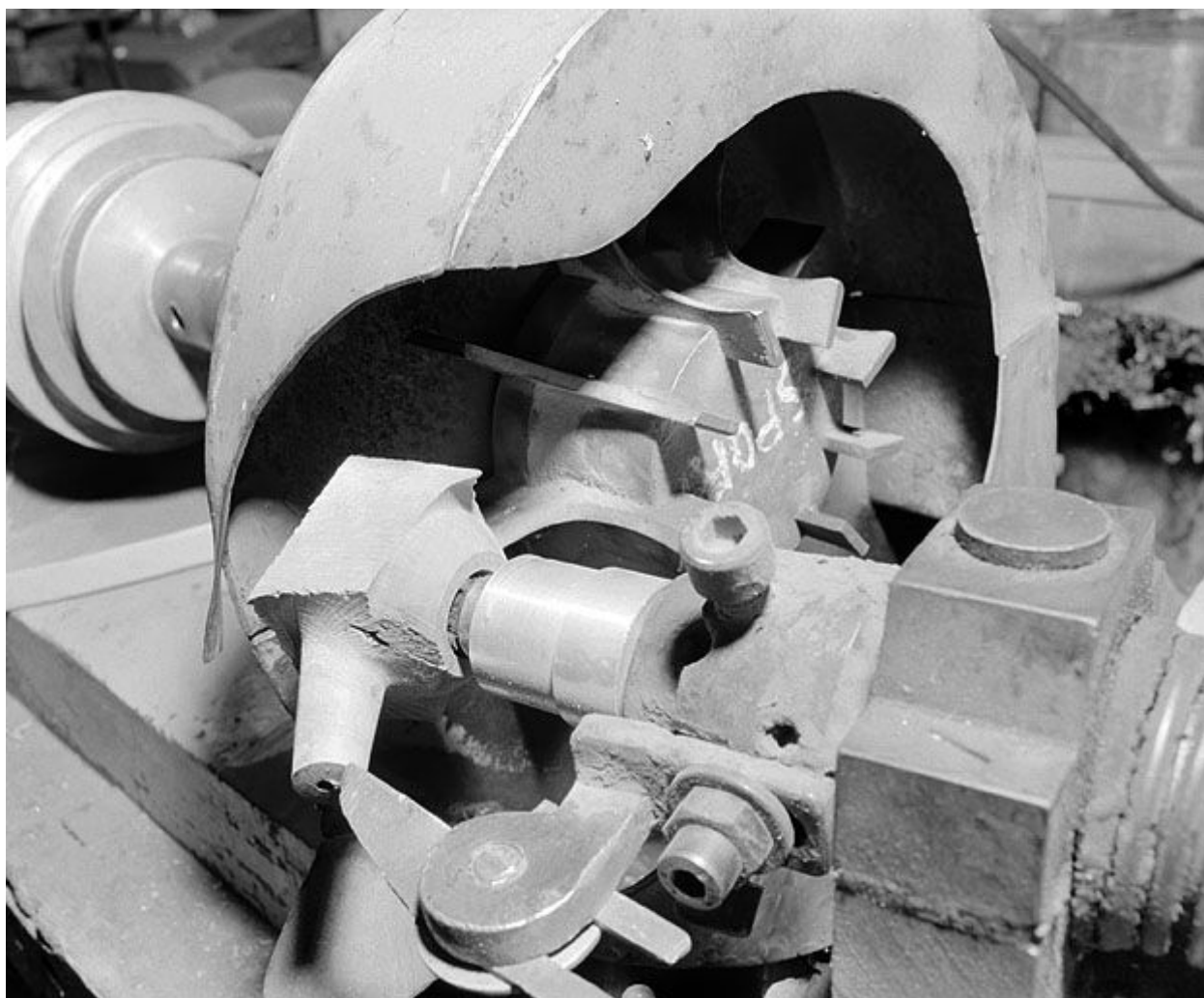
Mandrin conique et fraise.
