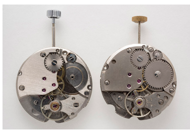
Deux mouvements de montre mécaniques France Ebauches FE 140-1 et 140-2A.
