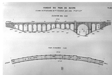
Viaduc du Pain de Sucre à 1 arche de 15 m et 15 arches de 5 m d'ouverture plein-cintre. Plan d'ensemble [et] Elévation aval, [1919]. Phot. Jérôme Mongreville IVR43_20003900903X
