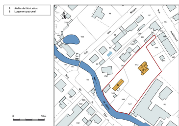
Plan-masse et de situation. Dess. Mathias Papigny IVR43_20132502607NUDA
