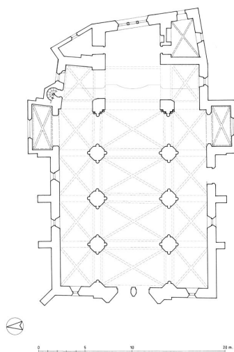
Plan. Dess. Alain Morelière IVR26_20128900020A2YY
