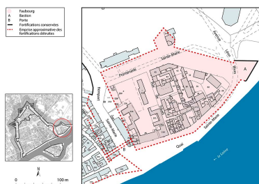
Plan-masse et de situation. Extrait du plan cadastral, 2025, 1/2 000. Dess. Aline Thomas IVR26_20257100358NUDA
