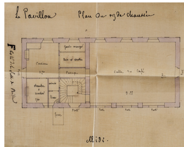
Le Pavillon, plan du rez-de-chaussée. Phot. Pierre-Marie Barbe-Richaud, Autr. auteur inconnu IVR26_20195800330NUC2A
