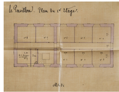
Le Pavillon, plan du premier étage. Phot. Pierre-Marie Barbe-Richaud, Autr. auteur inconnu IVR26_20195800331NUC2A
