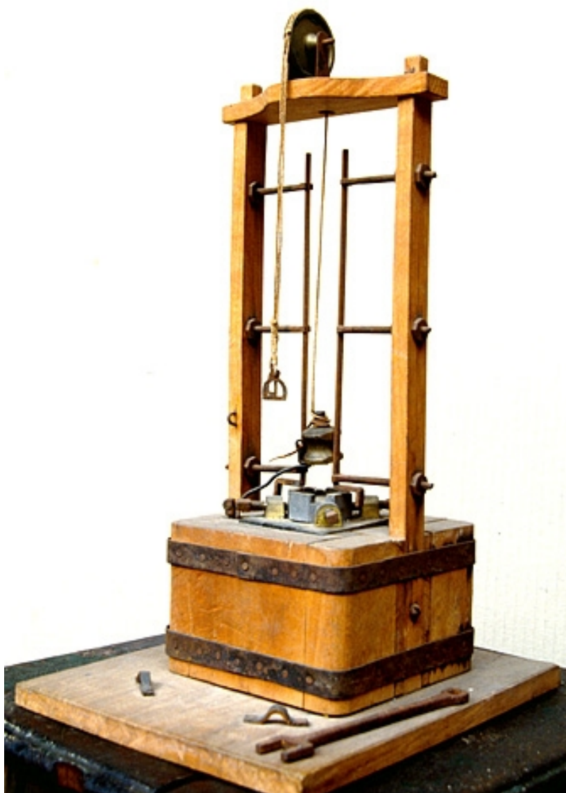
Mouton servant autrefois à l'estampage.
