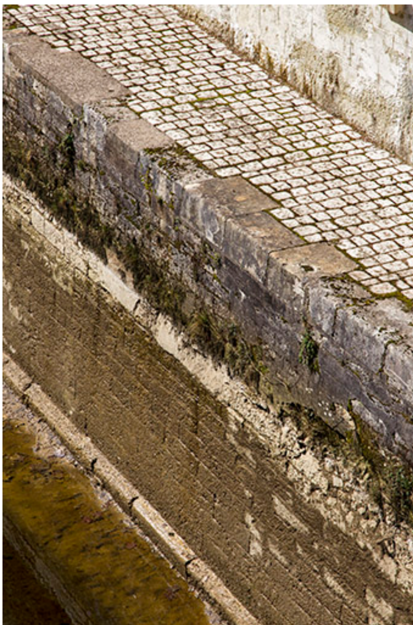
Banquette de halage, mur latéral canal et radier.
