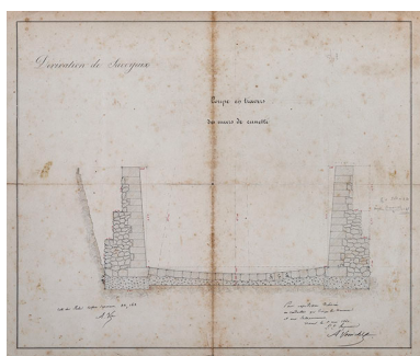
Dérivation de Savoyeux - coupe en travers des murs de cuvette (1840). Phot. Jérôme Mongreville, Autr. A. Voinchez IVR43_20207000106NUC4A
