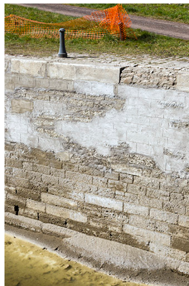
Détail de la maçonnerie lors des travaux de restauraton en 2015. Phot. Sonia Dourlot IVR43_20157000255NUC2A
