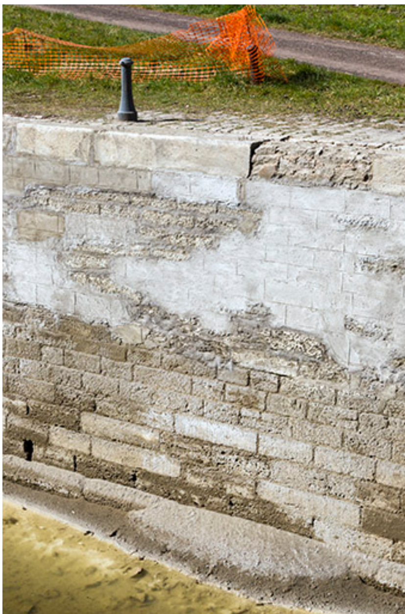
Détail de la maçonnerie lors des travaux de restauraton en 2015.
