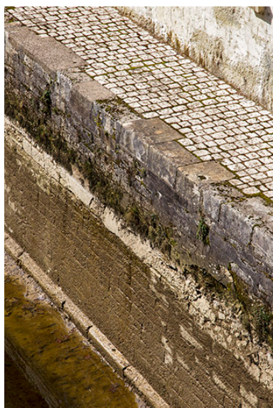
Banquette de halage, mur latéral canal et radier. Phot. Sonia Dourlot IVR43_20157000254NUC2A
