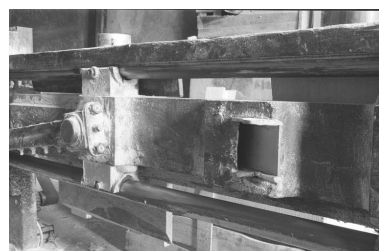
Targeuse : côté de sortie des lanières de bois. Phot. Laurent Poupard IVR43_19913901617Z
