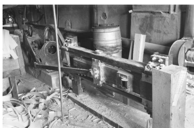
Vue d'ensemble de la targeuse, du côté de sortie des lanières de bois. Système moteur à gauche, rabot à droite. Phot. Laurent Poupard IVR43_19913901615Z
