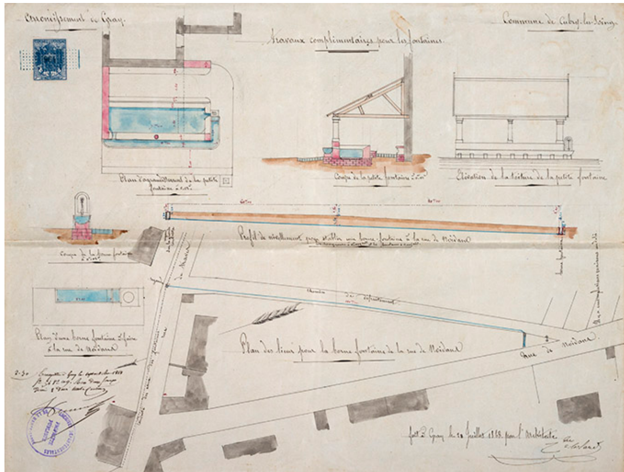
Travaux de la fontaine [Plans, coupes et élévations de la petite fontaine et de la borne-fontaine de la rue Noidans], 1868.
