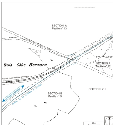
Plan-masse et de situation. Montage d'extraits du plan cadastral, 1995, sections A (12e feuille, 1:1250) et B (5e feuille, 1:2500), réduit à 1:3000. Dess. André Céréza IVR43_20073900194NUDA
