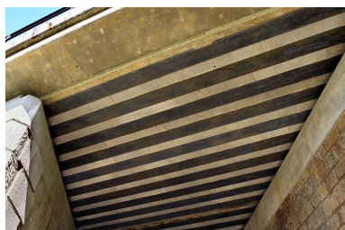
Face inférieure du tablier : poutres enrobées. Phot. Yves Sancey IVR43_20053900024ZA
