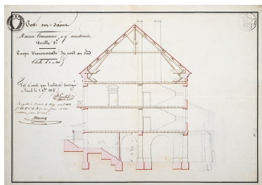
Coupe transversale du nord au sud (1836). Phot. Jérôme Mongreville, Autr. Jean-Baptiste Pambet IVR43_20177001156NUC4A
