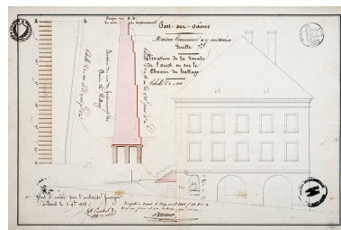
Elévation de la façade ouest (1836). Phot. Jérôme Mongreville, Autr. Jean-Baptiste Pambet IVR43_20177001154NUC4A
