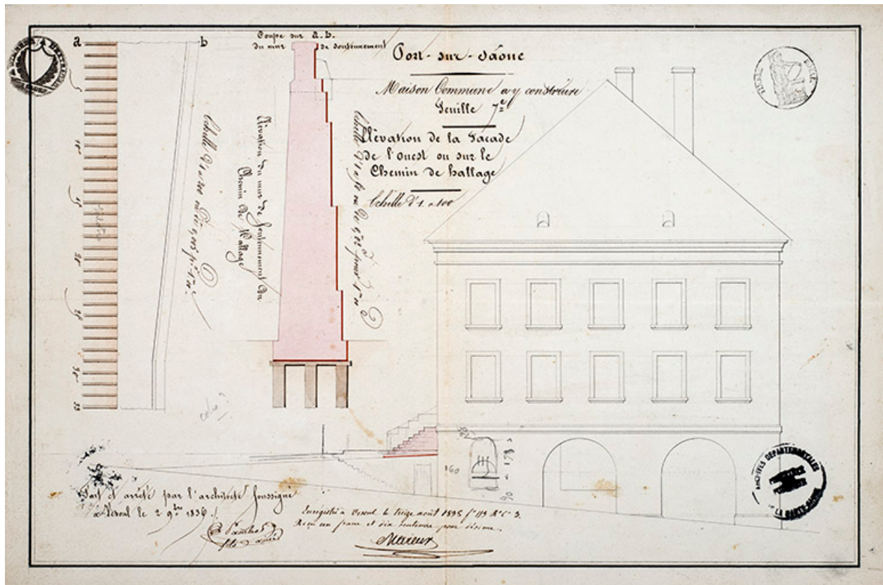
Elévation de la façade ouest (1836).
