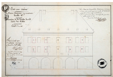
Plan de la façade du sud, entrée des halles (1836). Phot. Jérôme Mongreville, Autr. Jean-Baptiste Pambet IVR43_20177001157NUC4A
