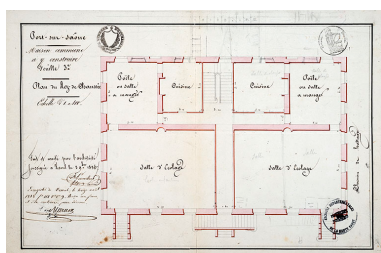
Plan du rez-de-chaussée (1836). Phot. Jérôme Mongreville, Autr. Jean-Baptiste Pambet IVR43_20177001152NUC4A
