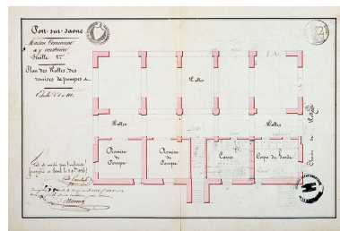
Plan de l'étage de soubassement (1836). Phot. Jérôme Mongreville, Autr. Jean-Baptiste Pambet IVR43_20177001158NUC4A
